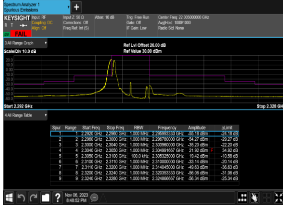
N30(5M)_DFT-s-OFDM_BPSK_Edge_1RB_Left_Low_CH
