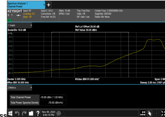
N30(5M)_DFT-s-OFDM_QPSK_Edge_1RB_Left_Low_CH_CHP_PA
