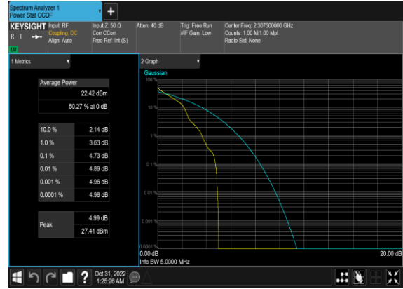
N30(5M)_DFT-s-OFDM_PI_2-BPSK_Edge_1RB_Left_ Low_CH
