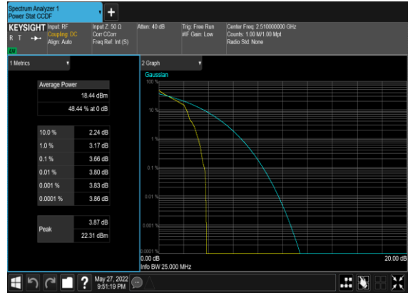
B2_N7(20M)_DFT-s-OFDM_PI_2-BPSK_Edge_1RB_Left_Low_CH
