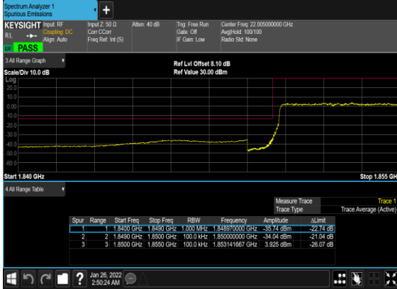
B66_N2(10M)_DFT-s-OFDM_BPSK_Outer_Full_Low_CH
