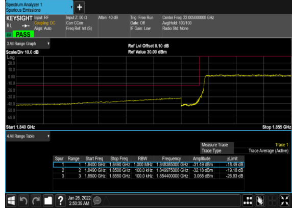
B66_N2(10M)_DFT-s-OFDM_QPSK_Outer_Full_Low_CH
