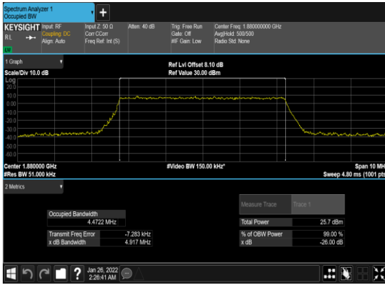
B66_N2(5M)_CP- OFDM_QPSK_Outer_Full_Mid_CH
