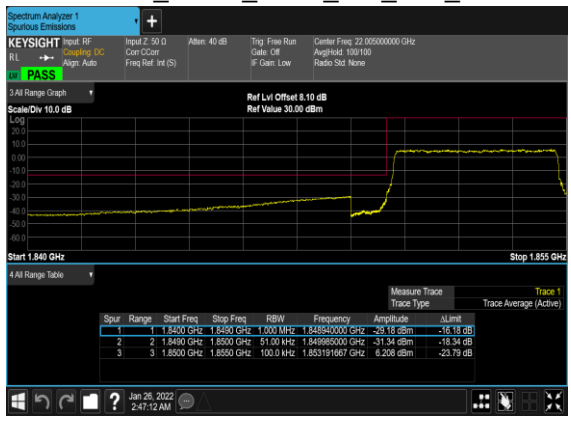
B66_N2(5M)_DFT-s-OFDM_QPSK_Outer_Full_Low_CH
