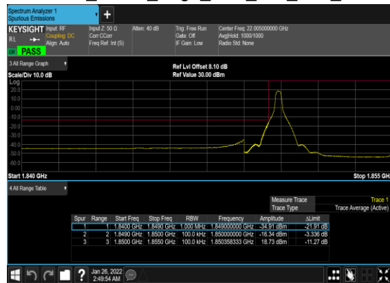
B66_N2(10M)_DFT-s-OFDM_QPSK_Edge_1RB_Left_Low_CH
