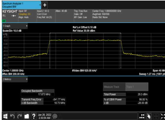
B66_N2(20M)_DFT-s-OFDM_PI_2- BPSK_Outer_Full_Mid_CH
