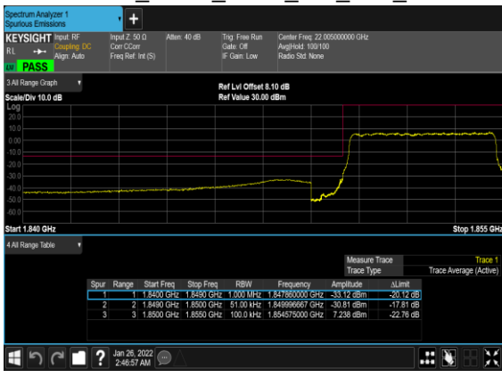
B66_N2(5M)_DFT-s-OFDM_BPSK_Outer_Full_Low_CH
