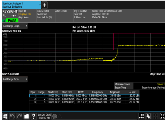
B66_N2(20M)_DFT-s-OFDM_BPSK_Outer_Full_Low_CH
