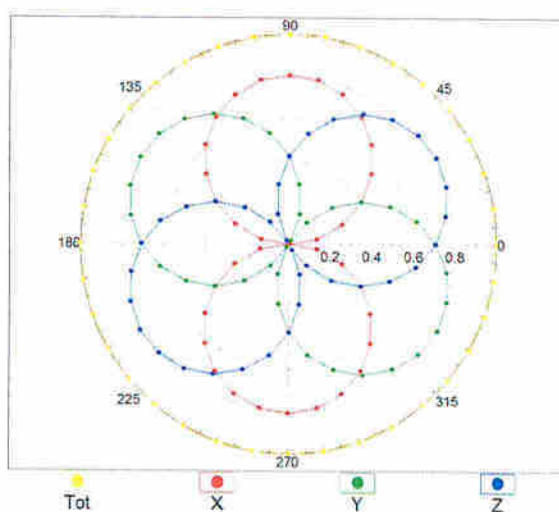
f=1800 MHz,R22
