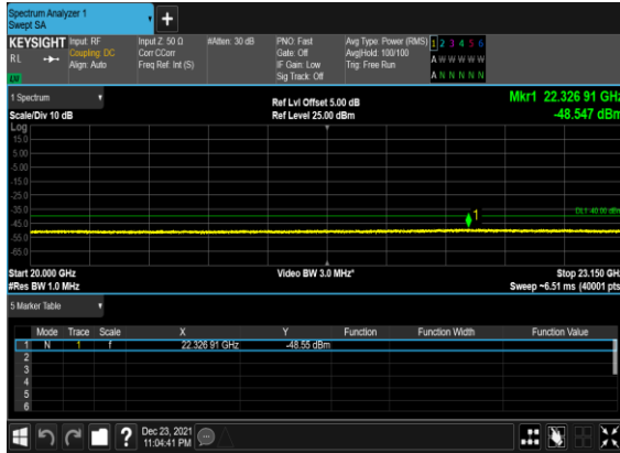
B2_N30(5M)_DFT-s-OFDM_BPSK_Edge_1RB_Left_Low_CH
