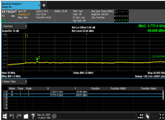
B2_N30(5M)_DFT-s-OFDM_QPSK_Edge_1RB_Left_Low_CH
