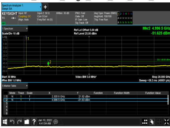
B2_N30(5M)_DFT-s-OFDM_BPSK_Edge_1RB_Left_Low_CH
