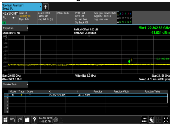
B2_N30(5M)_DFT-s-OFDM_BPSK_Edge_1RB_Left_Low_CH
