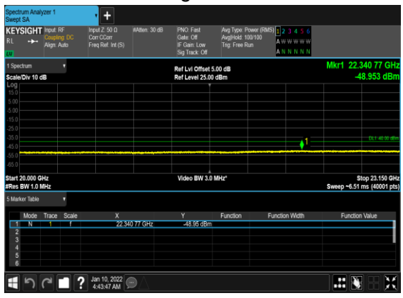
B2_N30(5M)_DFT-s-OFDM_QPSK_Edge_1RB_Left_Low_CH
