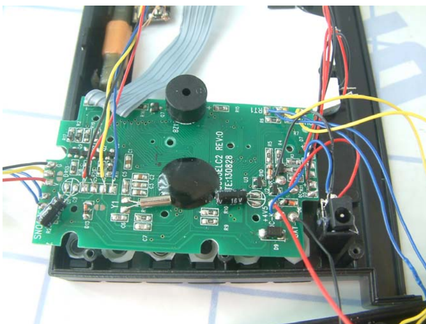
PCB 1 side2
