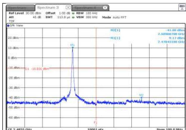
Result of 2 483.5 MHz (F1 : 2 483.5 MHz)
