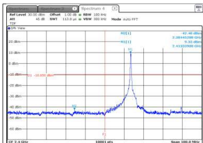
Result of 2 400.0 MHz (F1 : 2 400 MHz)
