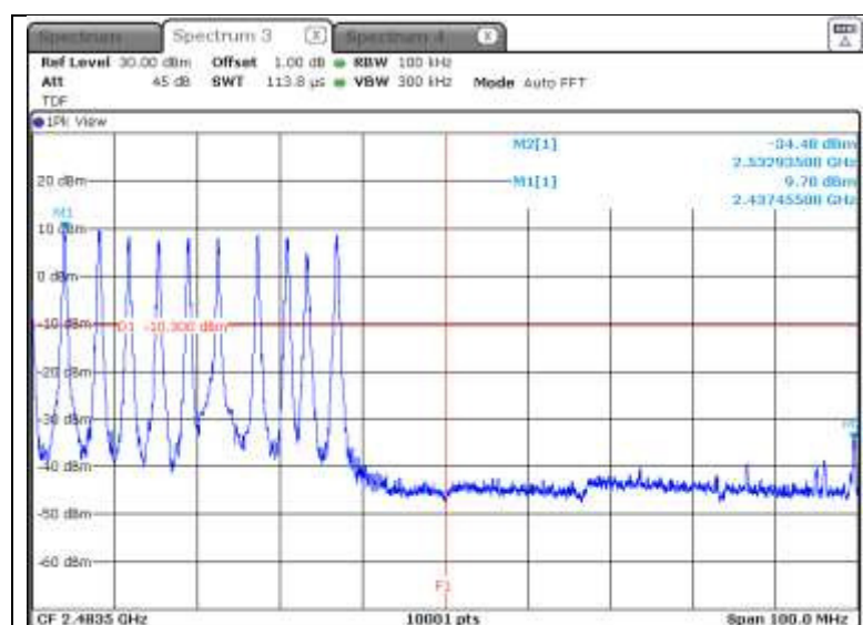
Result of 2 483.5 MHz (F1 : 2 483.5 MHz)
