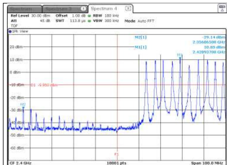
Result of 2 400.0 MHz (F1 : 2 400 MHz)
