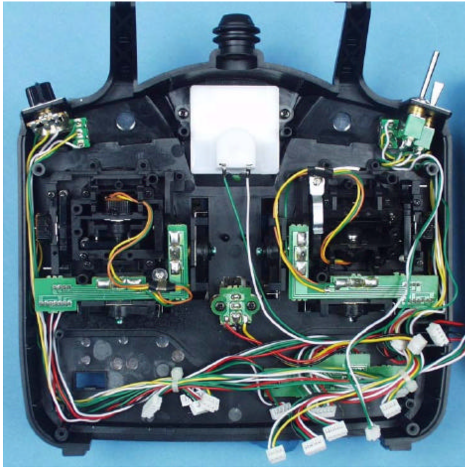
Internal, Wiring
