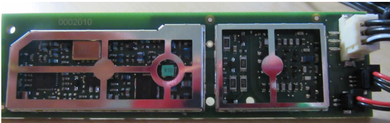
IDI-VLU10 Transciever PCB Bottom
