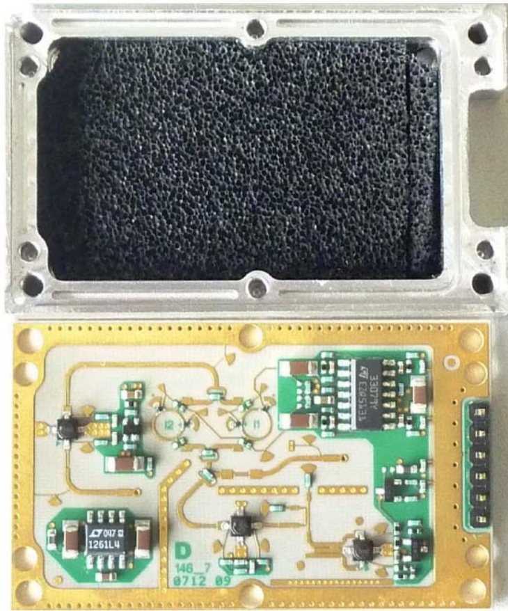
Microwave module 014-0007-00
