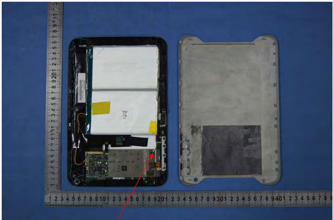
GPS Antenna
