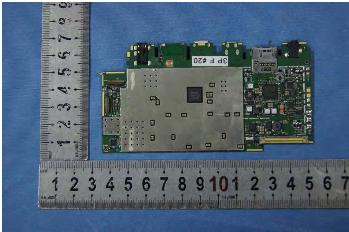
GPS module
