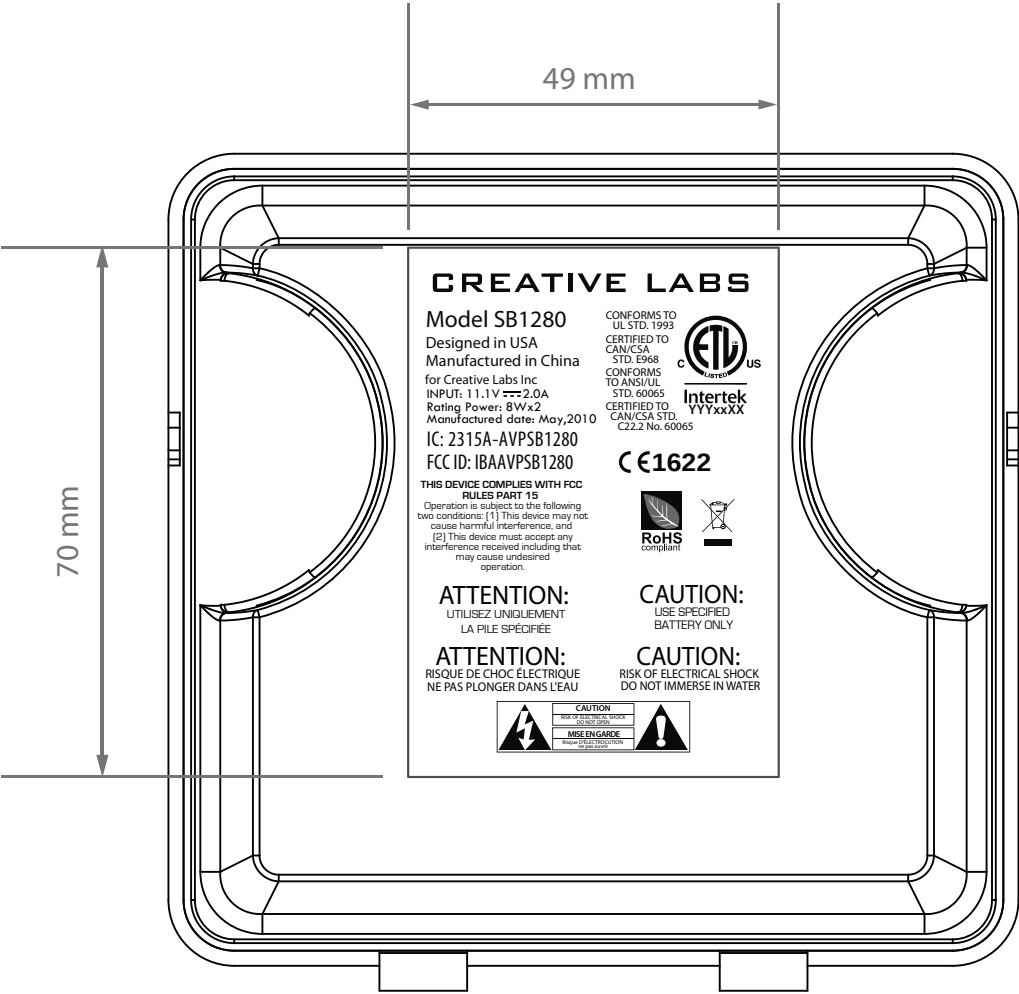
Label Dimensions
