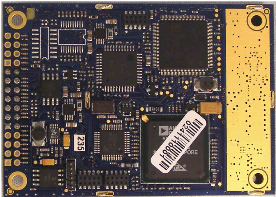
6.2 MR-900 Transceiver Module Bottom side:
