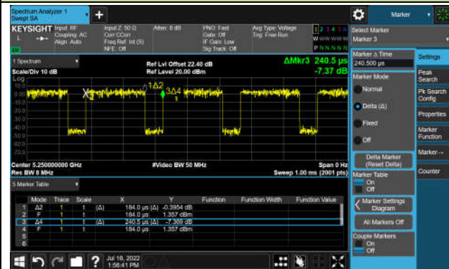
802.11ax-HE40 (T = 547.4µs)
