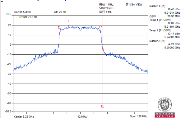
802.11ac(VHT40)_Chain2 / CH46
