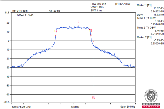
802.11a_Chain1 / CH48
