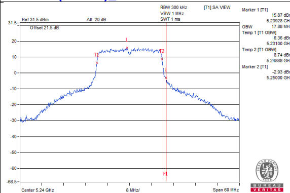
802.11ac(VHT20)_Chain1 / CH48
