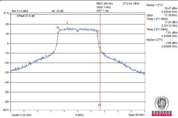
802.11ac(VHT20)_Chain2 / CH48
