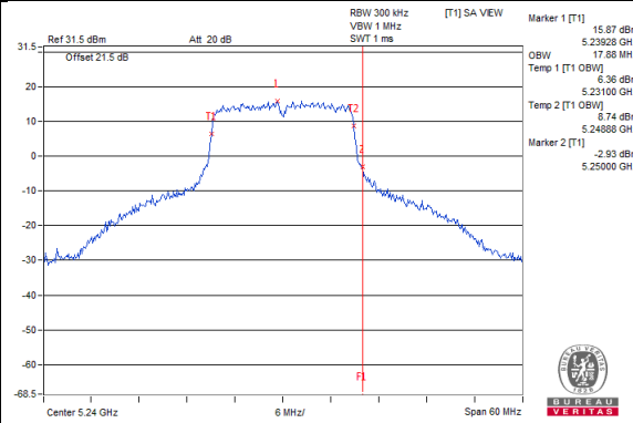
802.11ac(VHT20)_Chain1 / CH48
