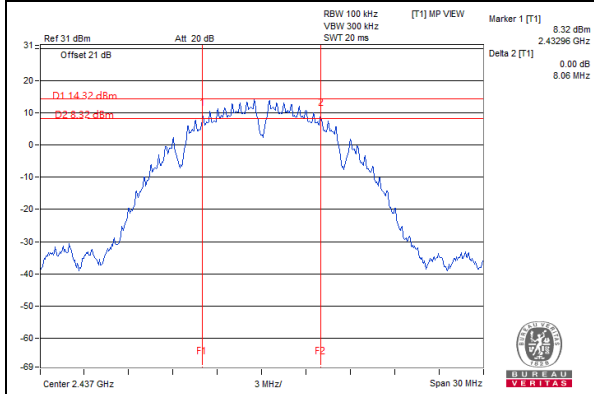
802.11ax (HE20) CDD \ Chain0 : CH 6
