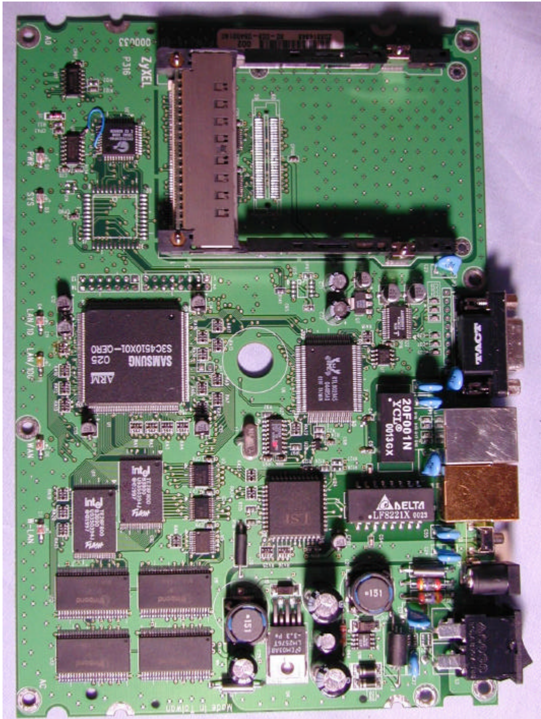
(4) EUT photo
