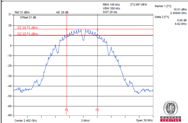
802.11ax (HE20) / Chain 3 : CH11
