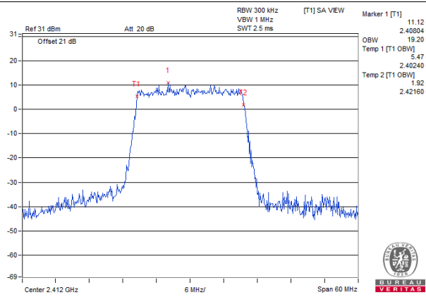
802.11ax (HE20)_Chain 0 / CH1
