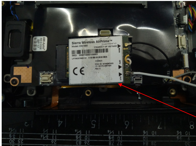
LTE Module
