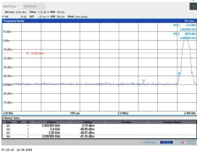
BLE_2M_Ant1_Low_2402
