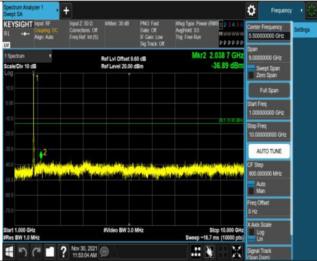
Band66-10MHz-QPSK-132322-50RB#0-Range2:1000~10000MHz
