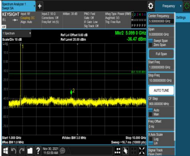
Band66-10MHz-QPSK-132622-50RB#0-Range2:1000~10000MHz
