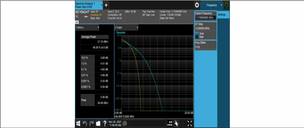
Band66-10MHz-QPSK-132022-50RB#0
