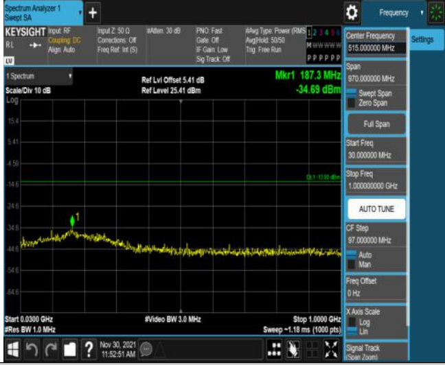
Band66-10MHz-QPSK-132322-50RB#0-Range1:30~1000MHz
