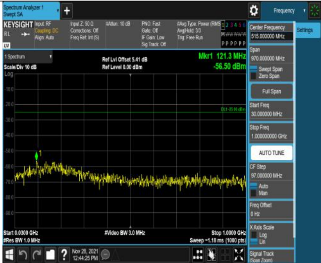
Band41-10MHz-QPSK-41540-50RB#0-Range1:30~1000MHz
