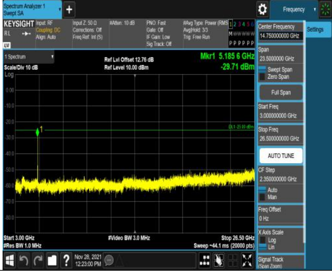
Band41-5MHz-QPSK-40620-25RB#0-Range3:3000~26500MHz
