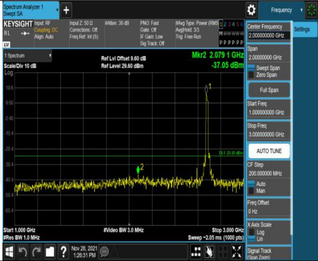
Band41-20MHz-QPSK-41490-100RB#0-Range2:1000~3000MHz
