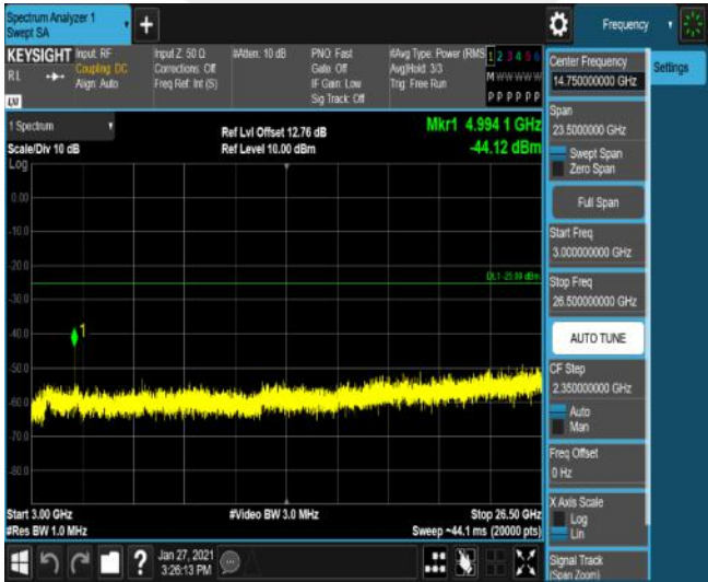
Band41-10MHz-16QAM-41540-50RB#0-Range3:3000~26500MHz
