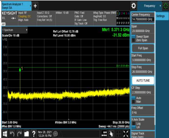
Band41-5MHz-QPSK-41565-25RB#0-Range3:3000~26500MHz
