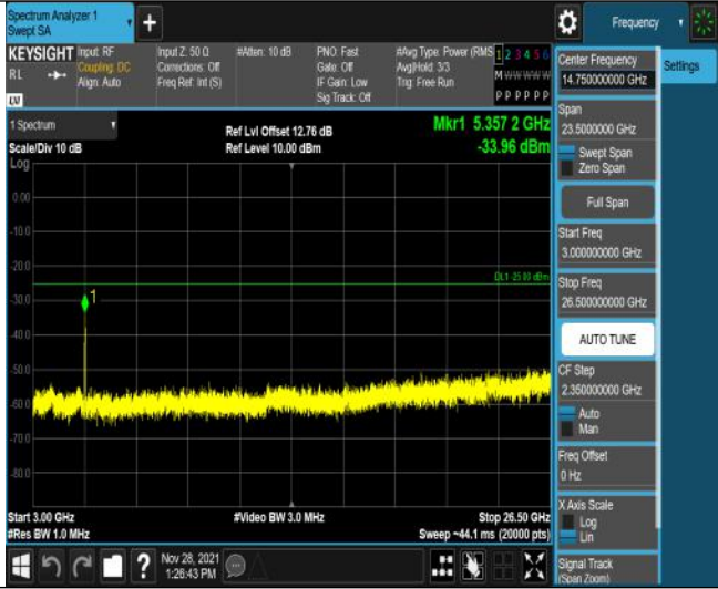
Band41-20MHz-QPSK-41490-100RB#0-Range3:3000~26500MHz
