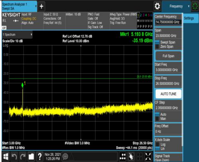
Band41-20MHz-QPSK-40620-100RB#0-Range3:3000~26500MHz
