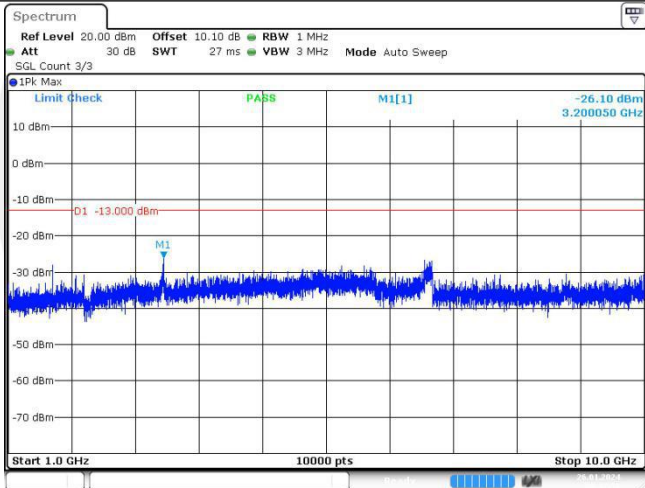
Band26-1.4MHz-QPSK-26697-1RB#0-Range2:1000~10000MHz
