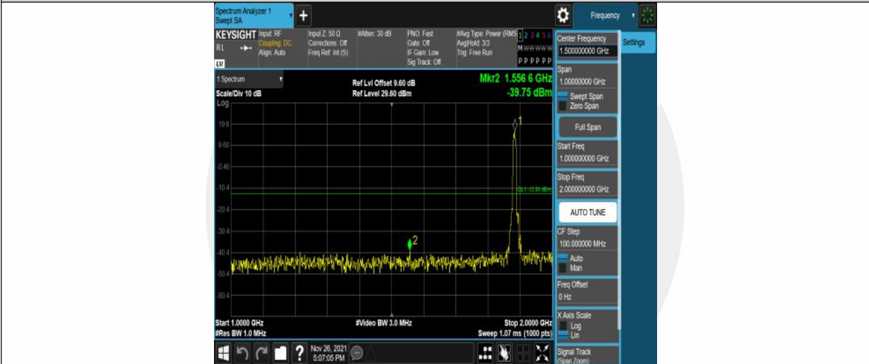
Band25-10MHz-16QAM-26365-50RB#0-Range2:1000~2000MHz
