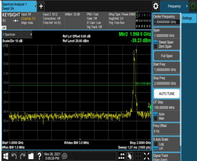
Band25-10MHz-QPSK-26365-50RB#0-Range2:1000~2000MHz
