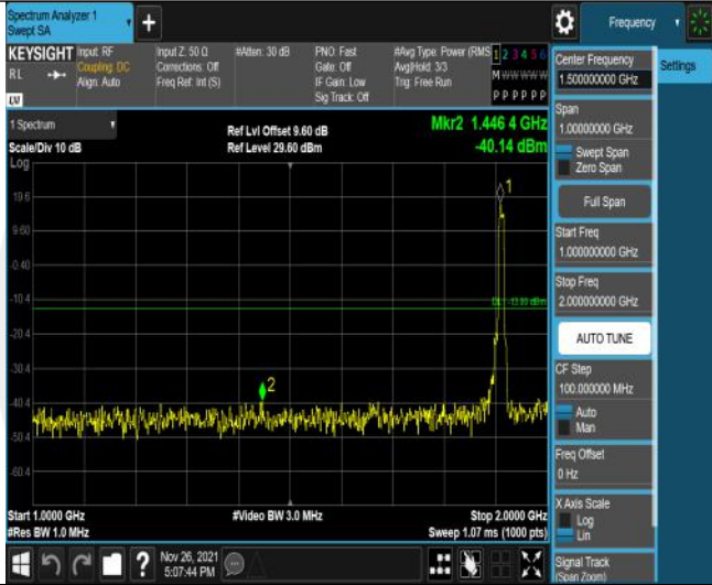
Band25-10MHz-QPSK-26640-50RB#0-Range2:1000~2000MHz
