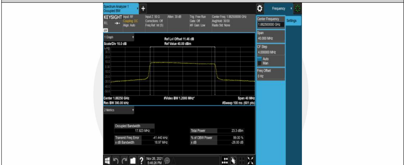
Band25-20MHz-QPSK-26365-100RB#0
