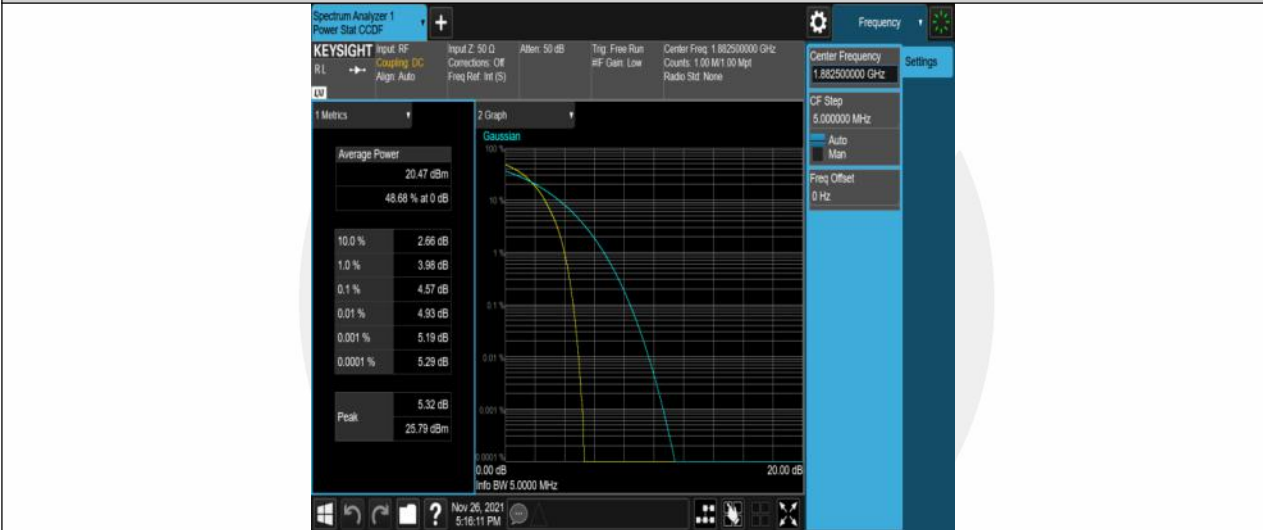
Band25-10MHz-QPSK-26365-50RB#0
