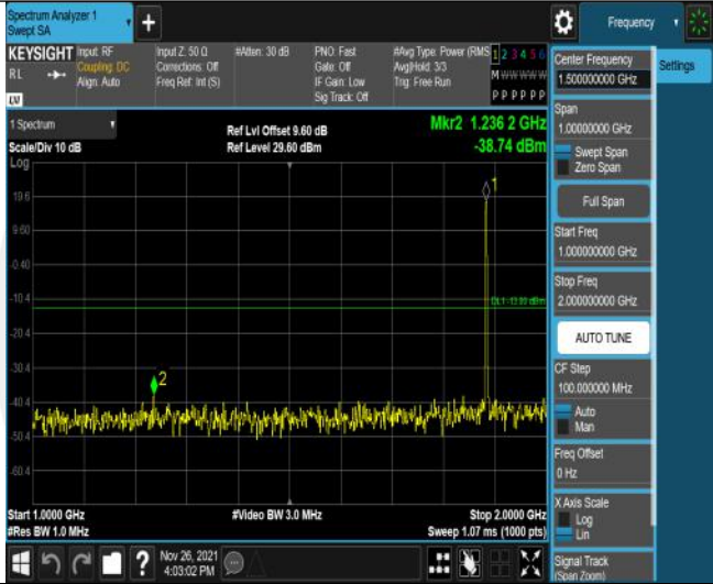
Band25-1.4MHz-16QAM-26365-6RB#0-Range2:1000~2000MHz
