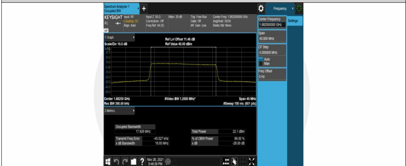
Band25-20MHz-16QAM-26365-100RB#0
