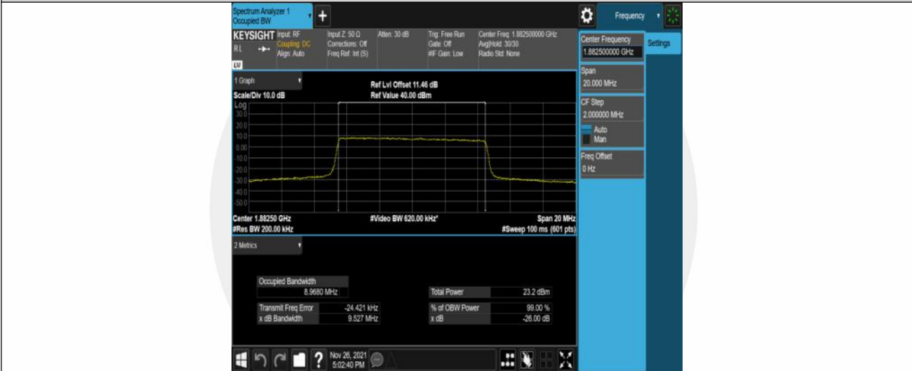
Band25-10MHz-QPSK-26365-50RB#0
