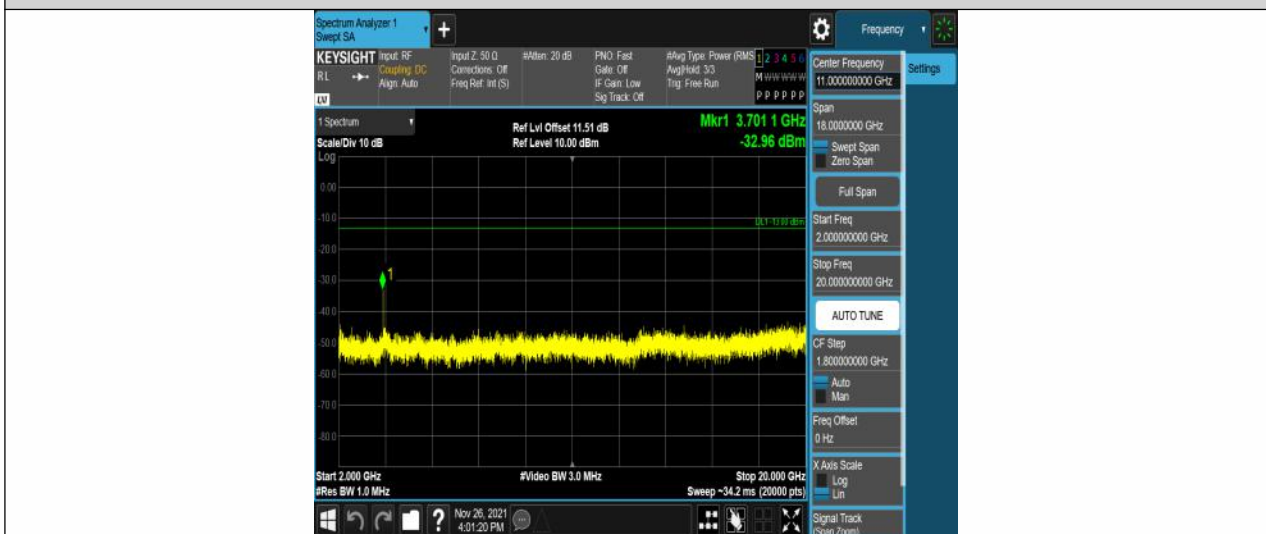
Band25-1.4MHz-QPSK-26047-6RB#0-Range3:2000~20000MHz
