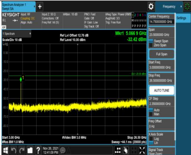
Band7-10MHz-QPSK-21100-50RB#0-Range3:3000~26500MHz
