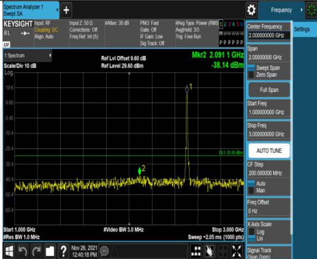
Band7-10MHz-16QAM-20800-50RB#0-Range2:1000~3000MHz
