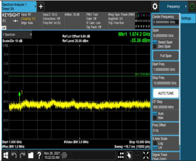
Band5-3MHz-QPSK-20525-15RB#0-Range2:1000~10000MHz
