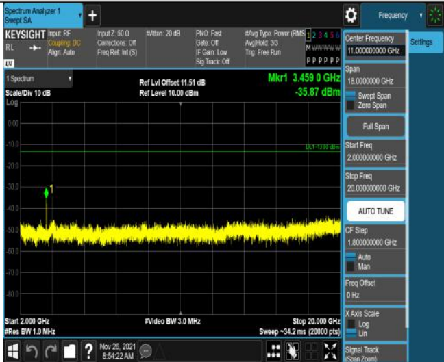
Band4-10MHz-QPSK-20175-50RB#0-Range3:2000~20000MHz
