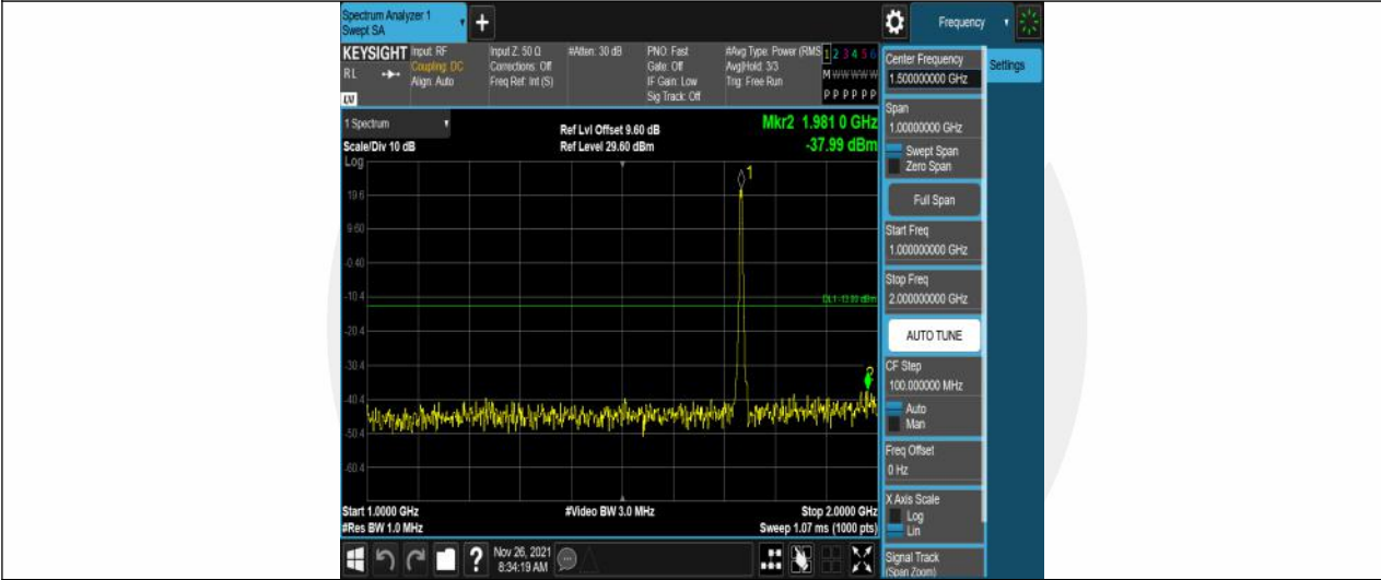
Band4-5MHz-QPSK-20175-25RB#0-Range2:1000~2000MHz
