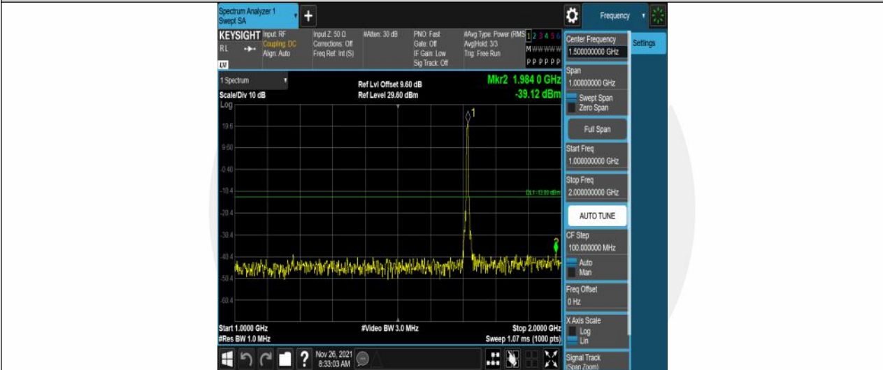
Band4-5MHz-QPSK-19975-25RB#0-Range2:1000~2000MHz
