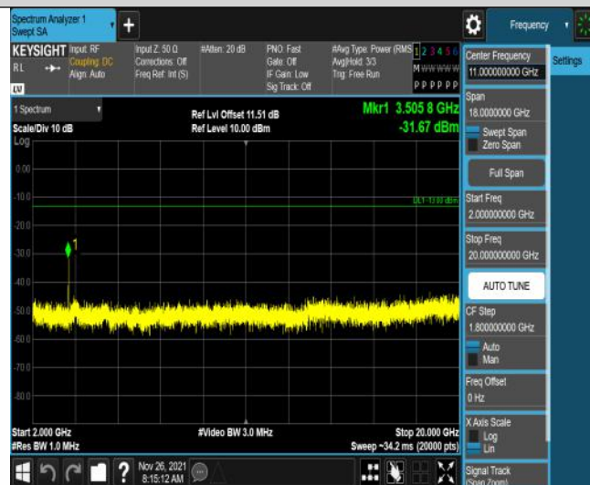
Band4-3MHz-QPSK-20385-6RB#0-Range3:2000~20000MHz
