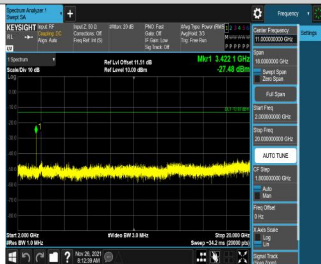
Band4-3MHz-QPSK-19965-6RB#0-Range3:2000~20000MHz
