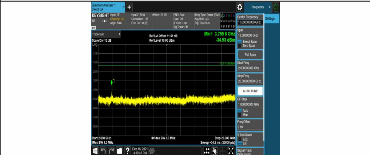
Band2-5MHz-QPSK-18900-25RB#0-Range3:2000~20000MHz
