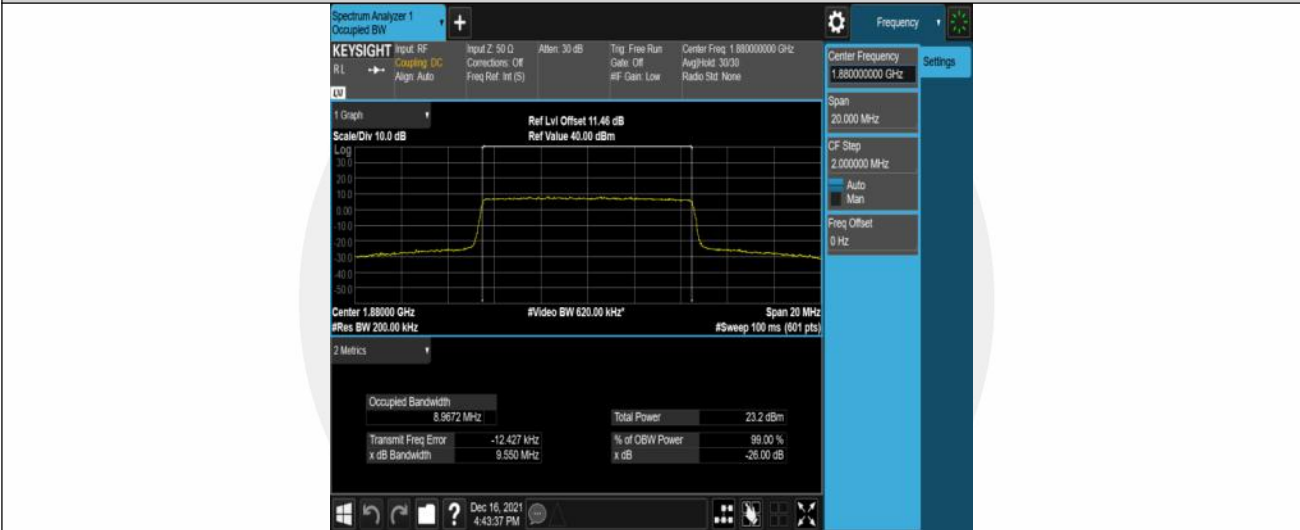
Band2-10MHz-16QAM-18900-50RB#0
