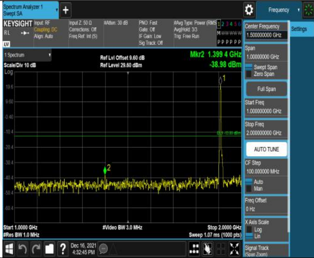
Band2-3MHz-QPSK-19185-15RB#0-Range2:1000~2000MHz
