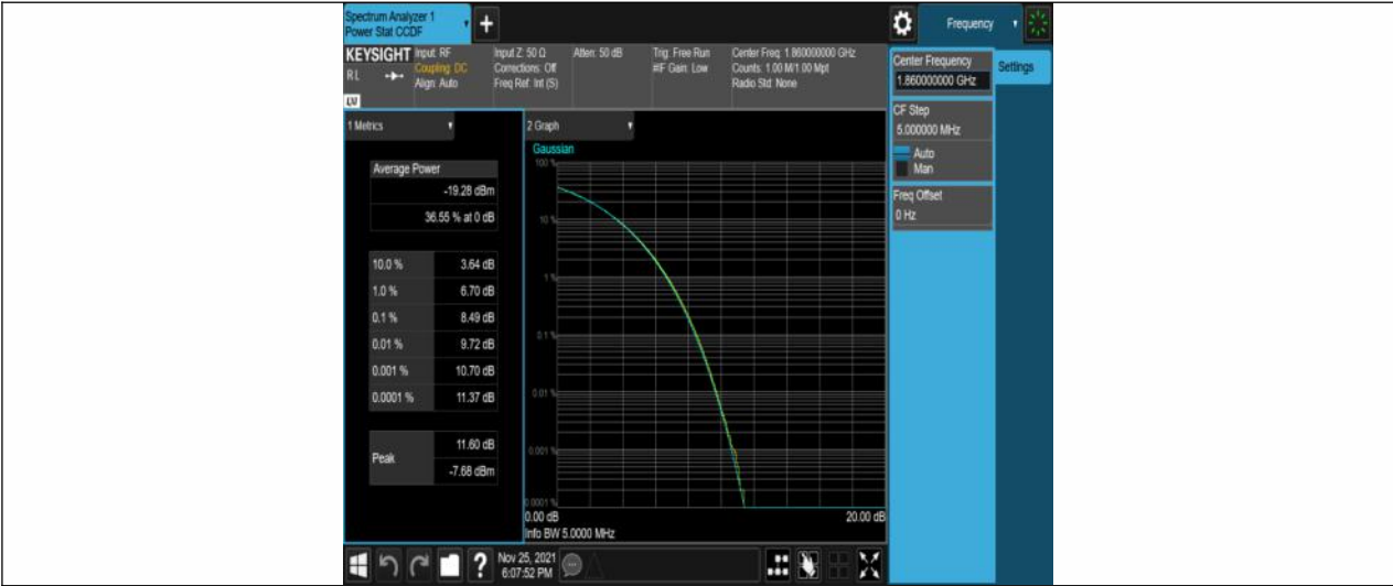
Band2-20MHz-16QAM-18700-100RB#0
