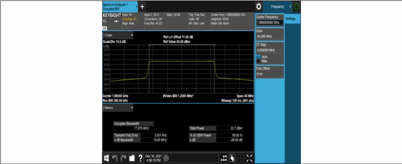
Band2-20MHz-16QAM-18700-100RB#0
