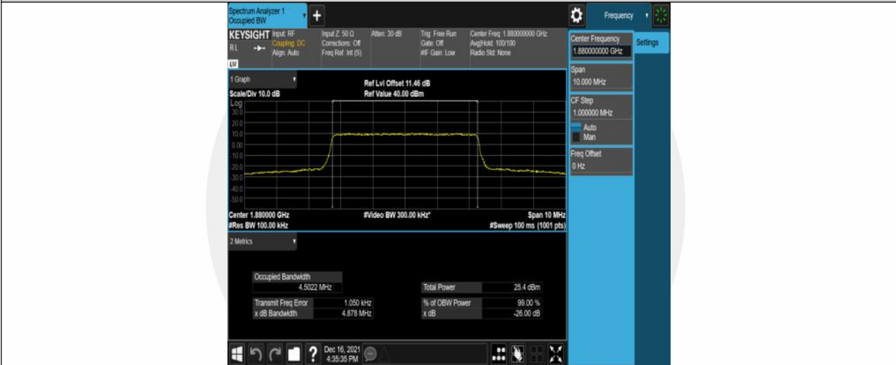
Band2-5MHz-QPSK-18900-25RB#0
