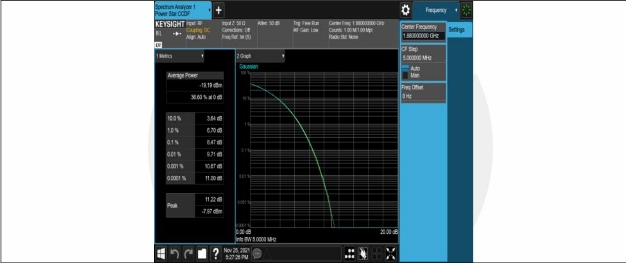
Band2-10MHz-16QAM-18900-50RB#0
