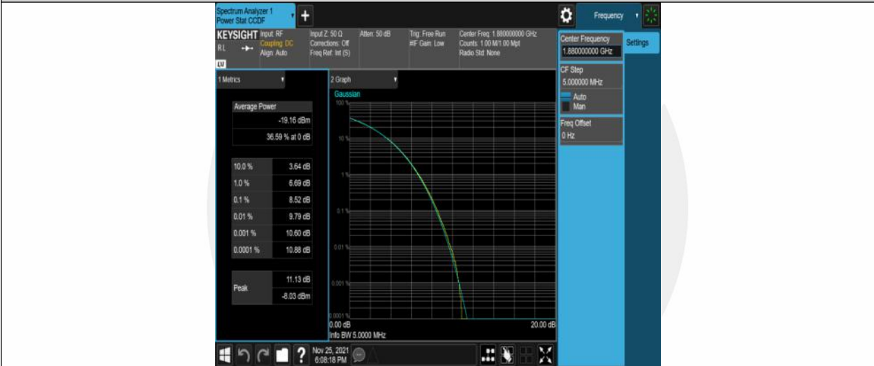
Band2-20MHz-16QAM-18900-100RB#0
