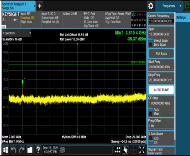
Band2-3MHz-QPSK-19185-15RB#0-Range3:2000~20000MHz
