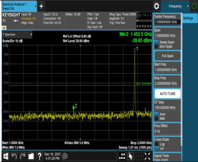
Band2-3MHz-QPSK-18900-15RB#0-Range2:1000~2000MHz
