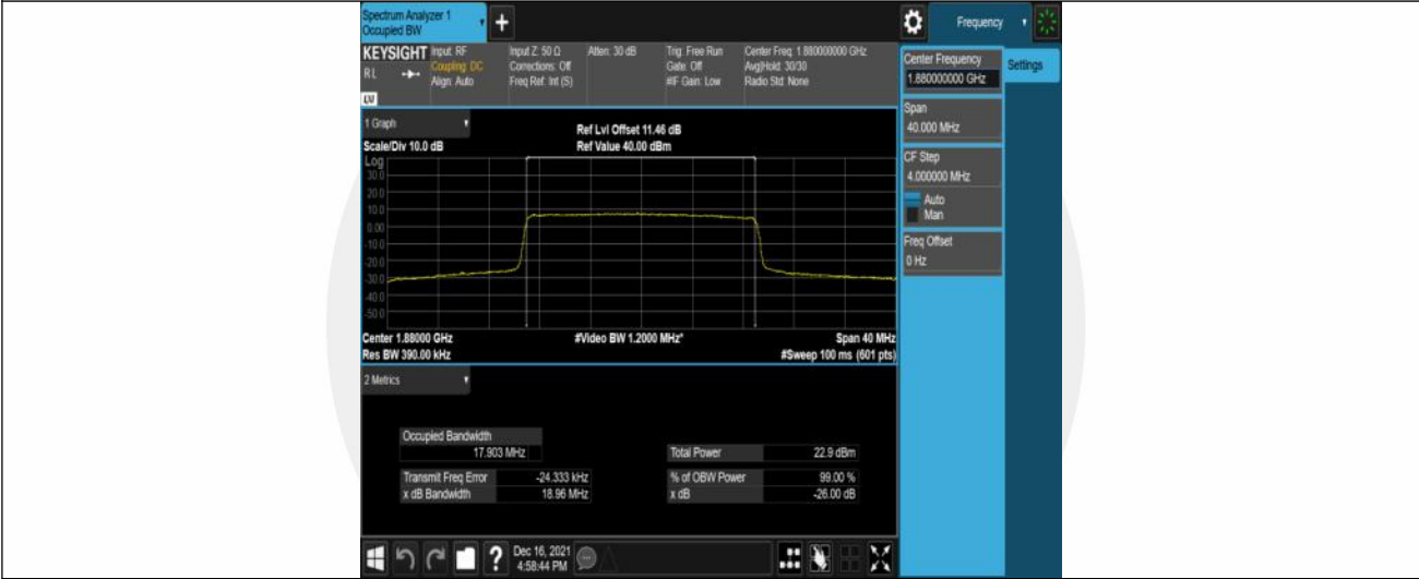
Band2-20MHz-16QAM-18900-100RB#0
