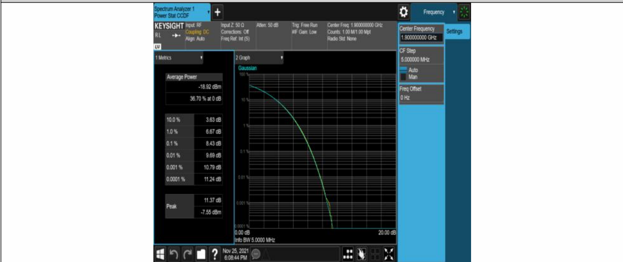
Band2-20MHz-16QAM-19100-100RB#0
