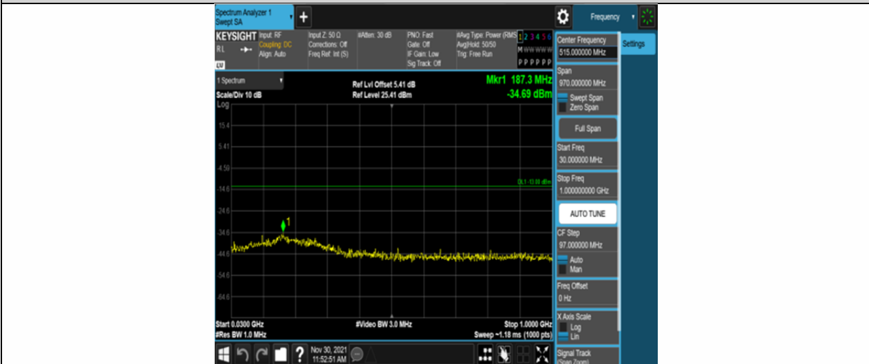
Band66-10MHz-QPSK-132322-50RB#0-Range1:30~1000MHz
