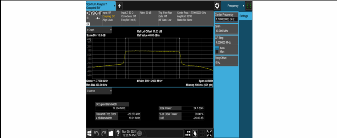
Band66-20MHz-QPSK-132572-100RB#0
