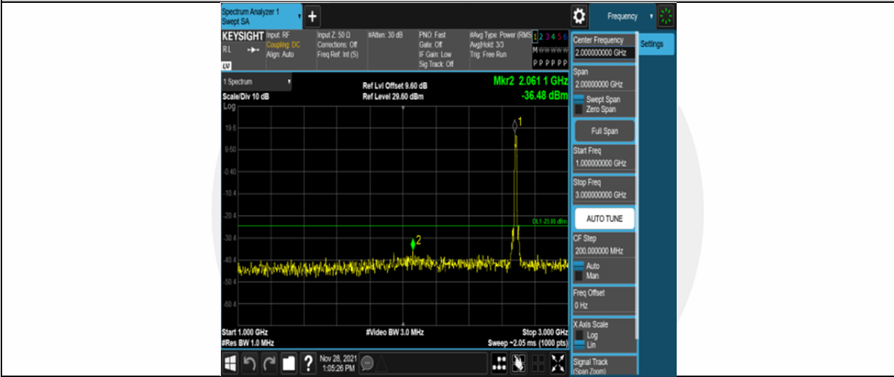
Band41-15MHz-QPSK-41515-75RB#0-Range2:1000~3000MHz
