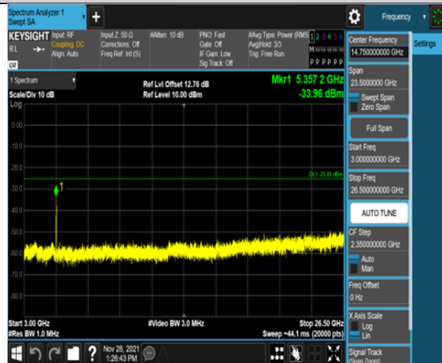
Band41-20MHz-QPSK-41490-100RB#0-Range3:3000~26500MHz
