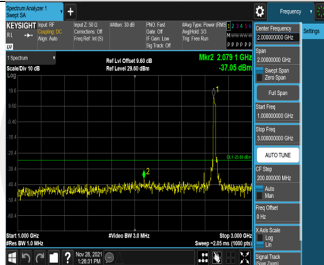
Band41-20MHz-QPSK-41490-100RB#0-Range2:1000~3000MHz
