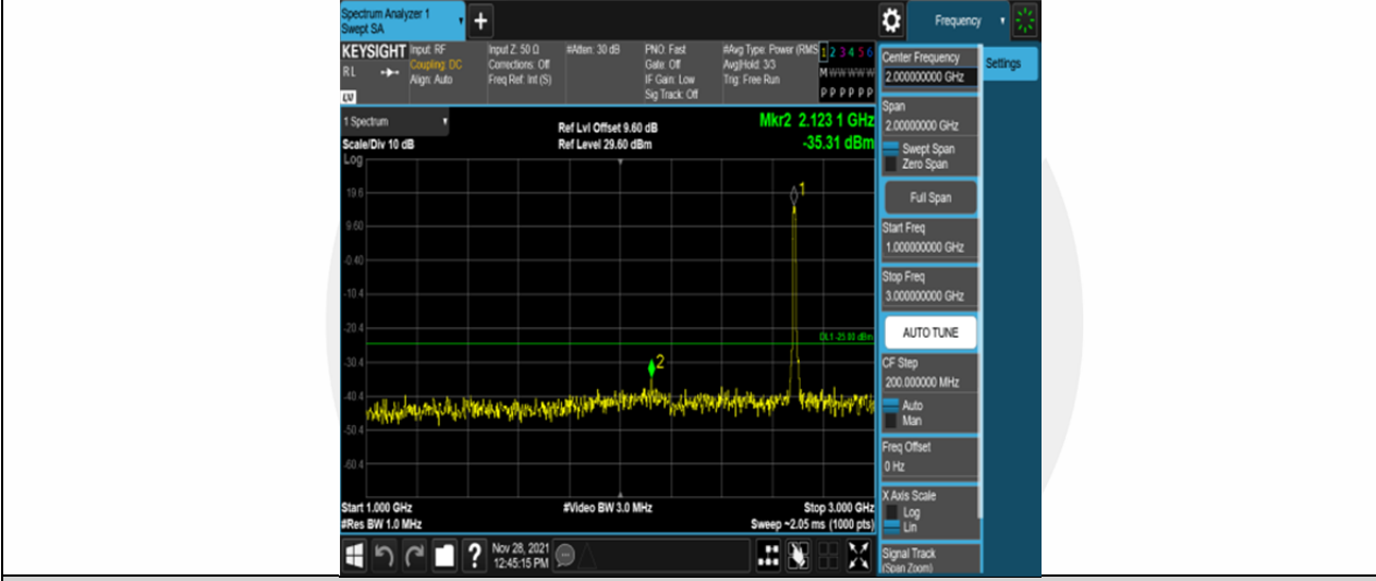
Band41-10MHz-16QAM-41540-50RB#0-Range2:1000~3000MHz
