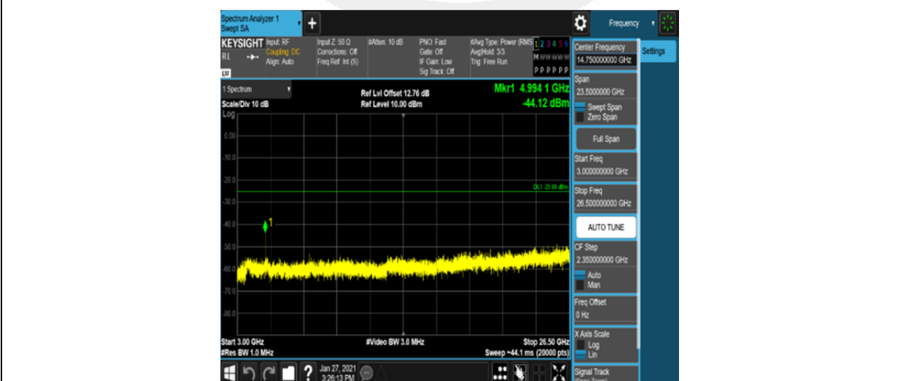
Band41-10MHz-16QAM-41540-50RB#0-Range3:3000~26500MHz
