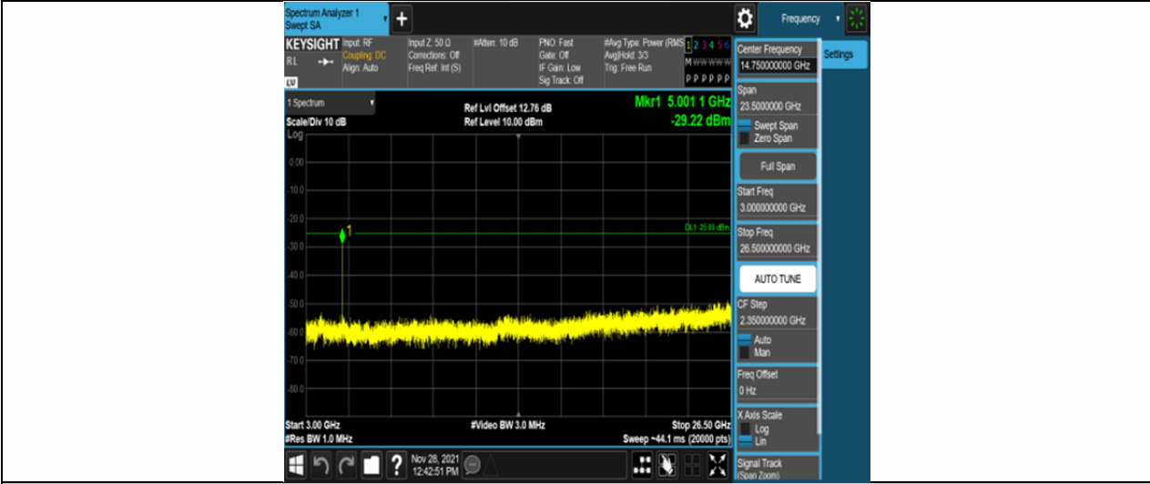
Band41-10MHz-16QAM-39700-50RB#0-Range3:3000~26500MHz
