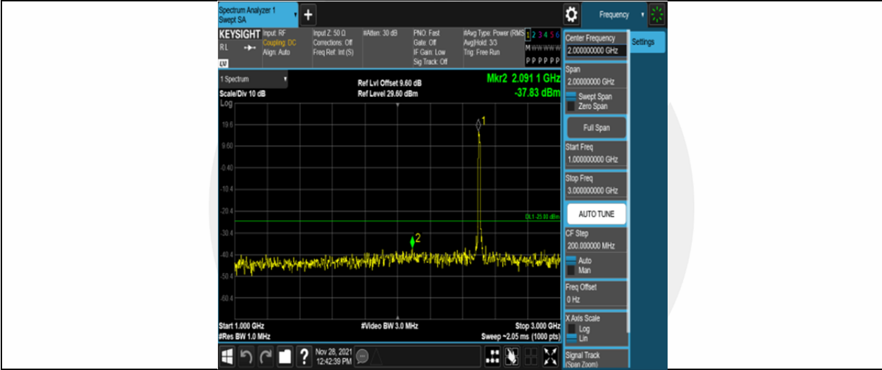
Band41-10MHz-16QAM-39700-50RB#0-Range2:1000~3000MHz
