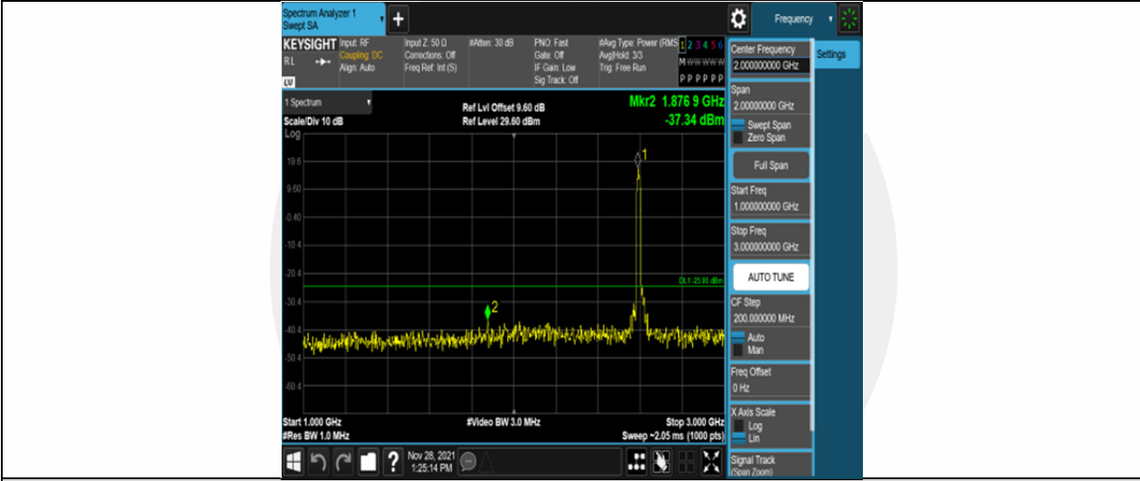
Band41-20MHz-QPSK-40620-100RB#0-Range2:1000~3000MHz
