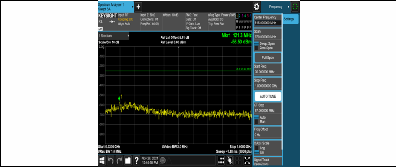
Band41-10MHz-QPSK-41540-50RB#0-Range1:30~1000MHz
