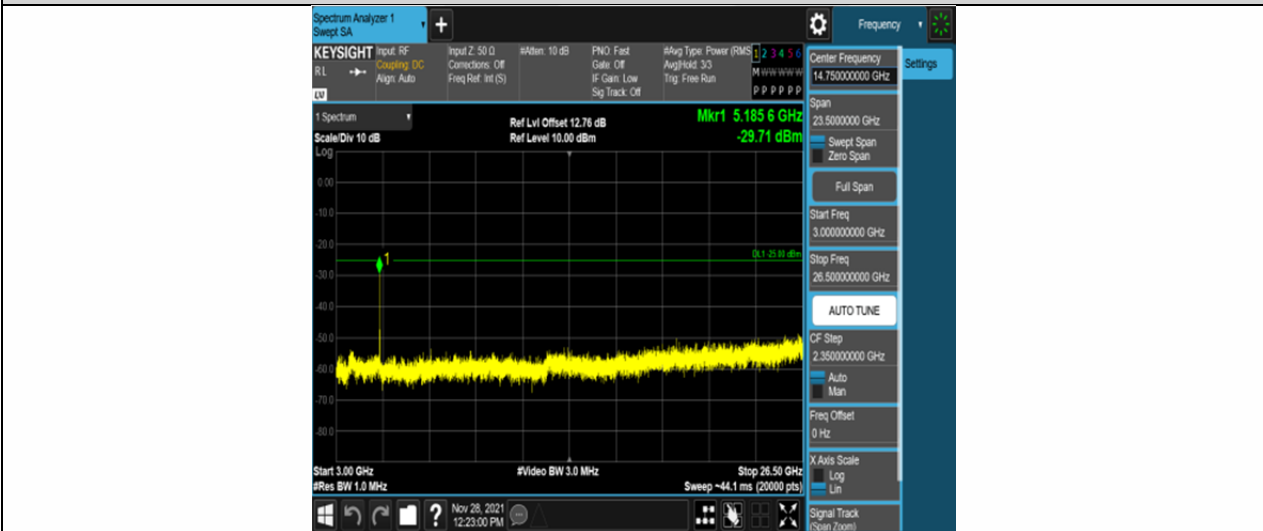
Band41-5MHz-QPSK-40620-25RB#0-Range3:3000~26500MHz
