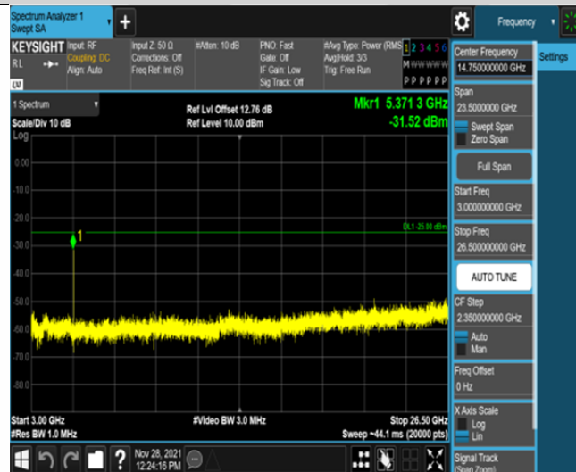
Band41-5MHz-QPSK-41565-25RB#0-Range3:3000~26500MHz
