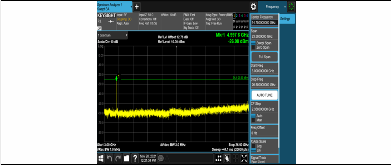
Band41-5MHz-QPSK-39675-25RB#0-Range3:3000~26500MHz
