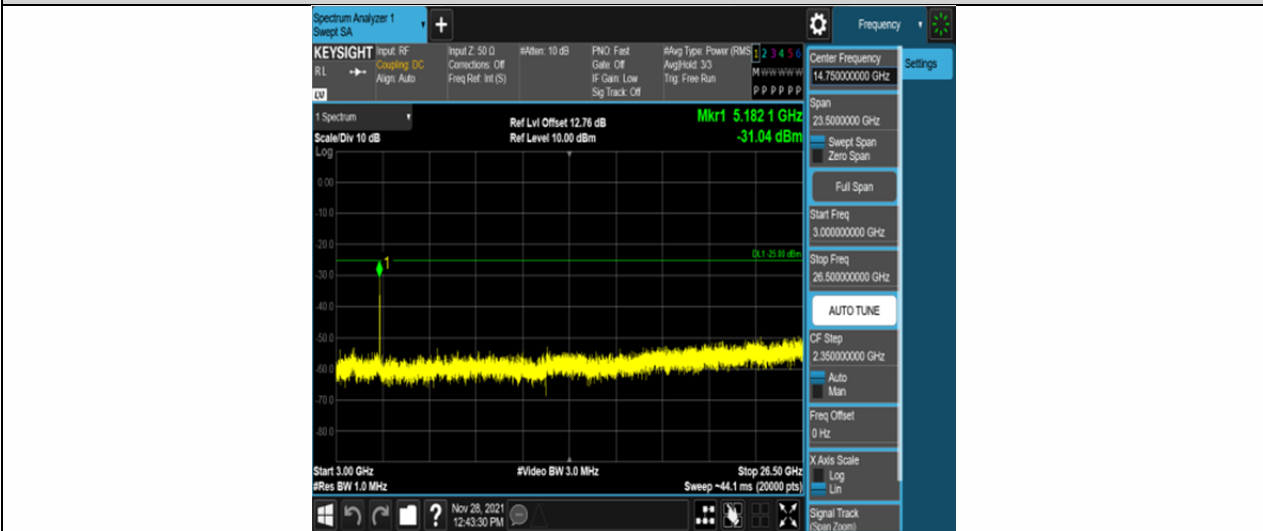
Band41-10MHz-QPSK-40620-50RB#0-Range3:3000~26500MHz
