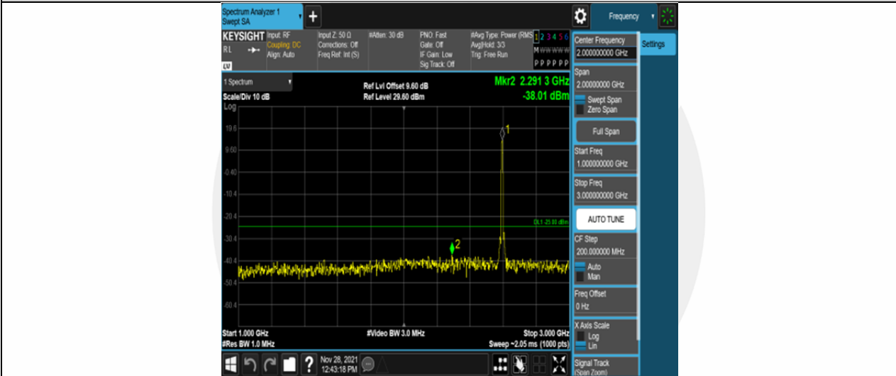
Band41-10MHz-QPSK-40620-50RB#0-Range2:1000~3000MHz
