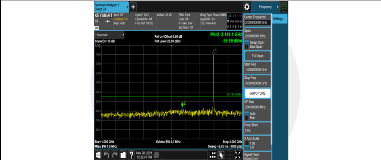
Band41-5MHz-QPSK-40620-25RB#0-Range2:1000~3000MHz
