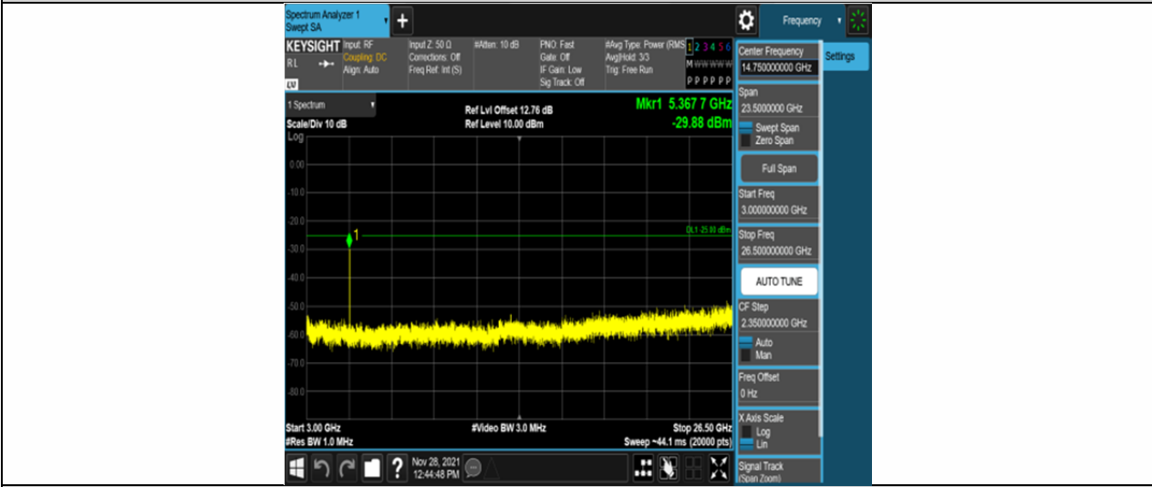
Band41-10MHz-QPSK-41540-50RB#0-Range3:3000~26500MHz
