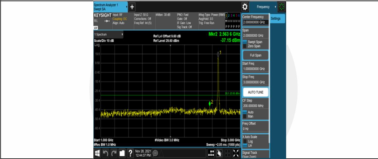
Band41-10MHz-QPSK-41540-50RB#0-Range2:1000~3000MHz
