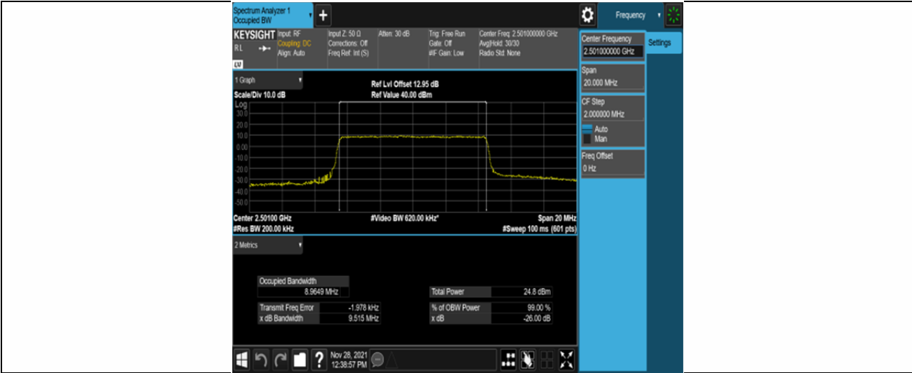
Band41-10MHz-QPSK-39700-50RB#0
