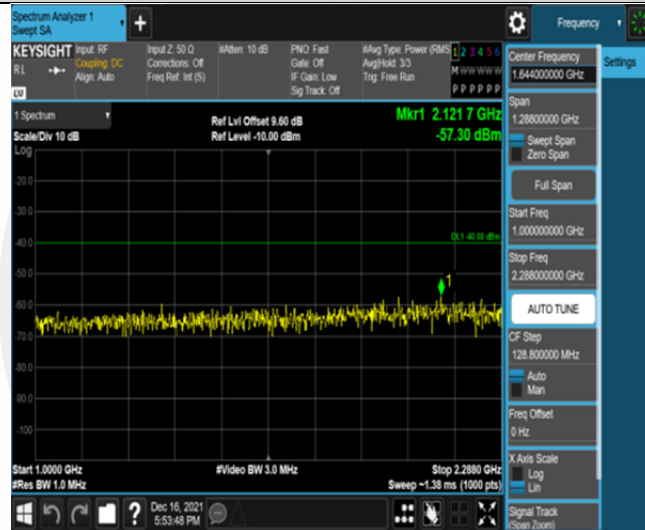
Band30-10MHz-QPSK-27710-50RB#0-Range2:1000~2288MHz
