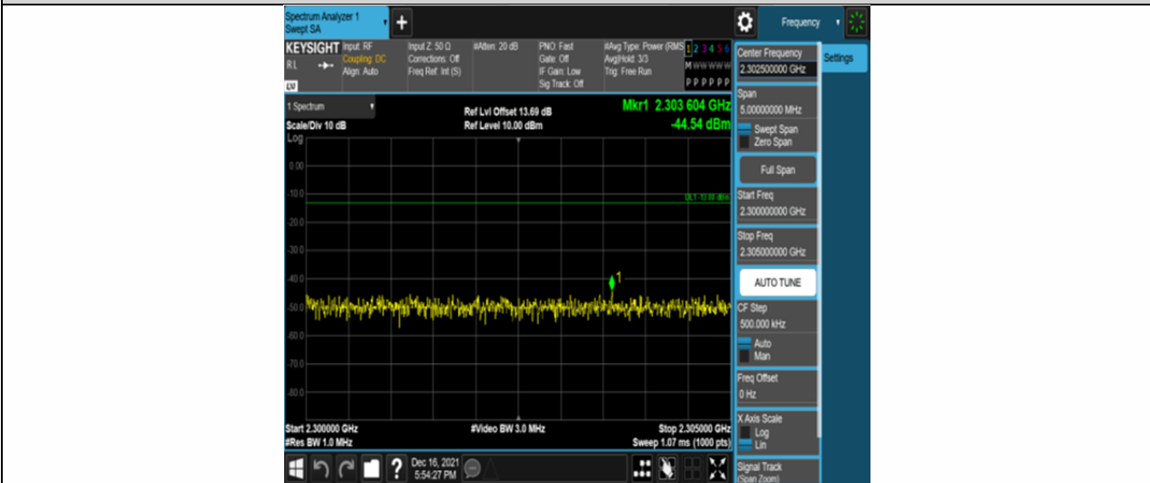
Band30-10MHz-QPSK-27710-50RB#0-Range6:2300~2305MHz
