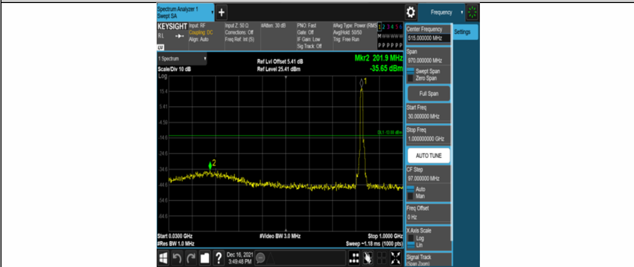
Band26-10MHz-QPSK-26840-50RB#0-Range1:30~1000MHz
