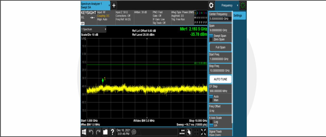
Band26-10MHz-QPSK-26990-50RB#0-Range2:1000~10000MHz
