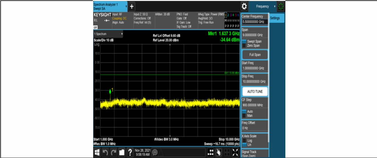
Band26-5MHz-QPSK-26740-25RB#0-Range2:1000~10000MHz
