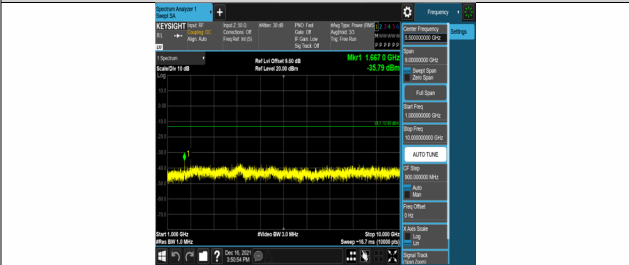
Band26-10MHz-QPSK-26915-50RB#0-Range2:1000~10000MHz
