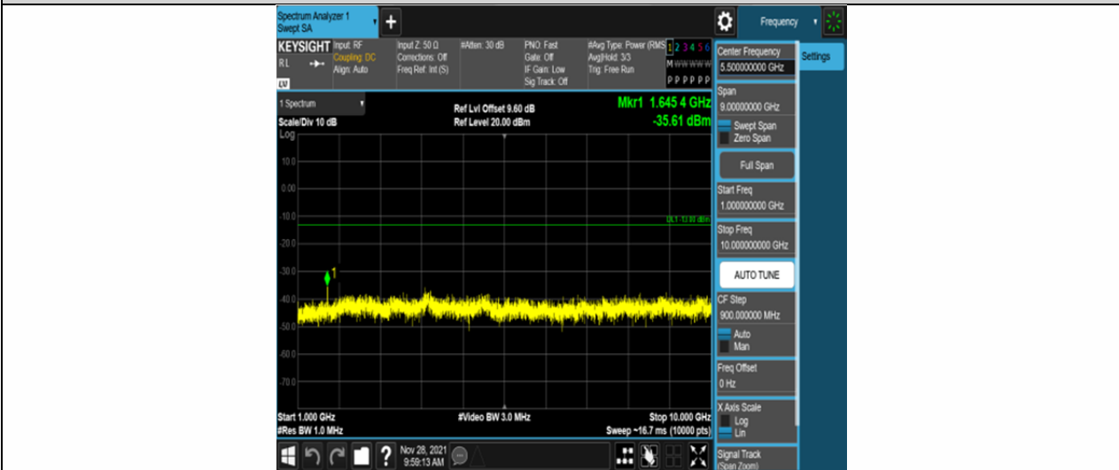
Band26-5MHz-QPSK-26765-25RB#0-Range2:1000~10000MHz
