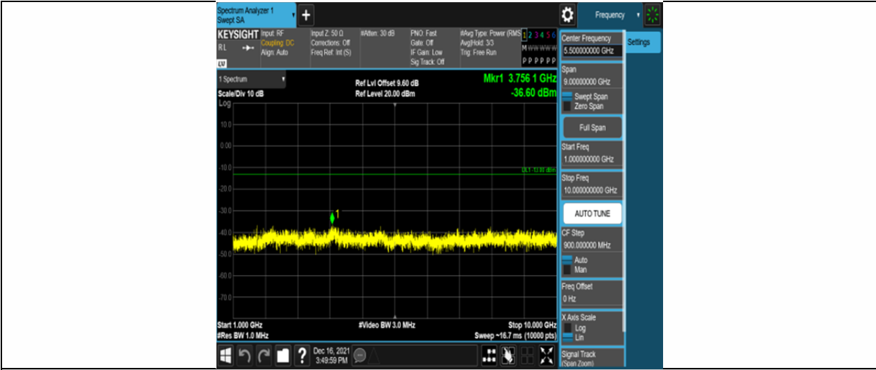
Band26-10MHz-QPSK-26840-50RB#0-Range2:1000~10000MHz
