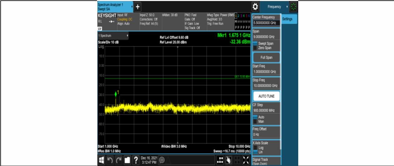
Band26-3MHz-QPSK-26915-15RB#0-Range2: 1000~10000MHz
