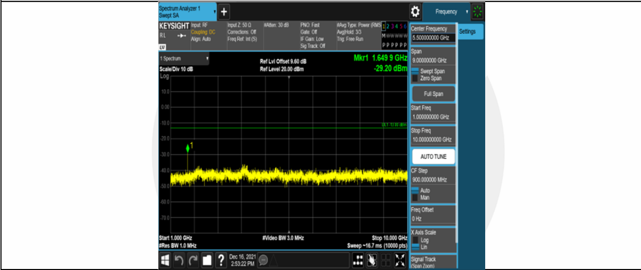
Band26-1.4MHz-QPSK-26797-6RB#0-Range2:1000~10000MHz
