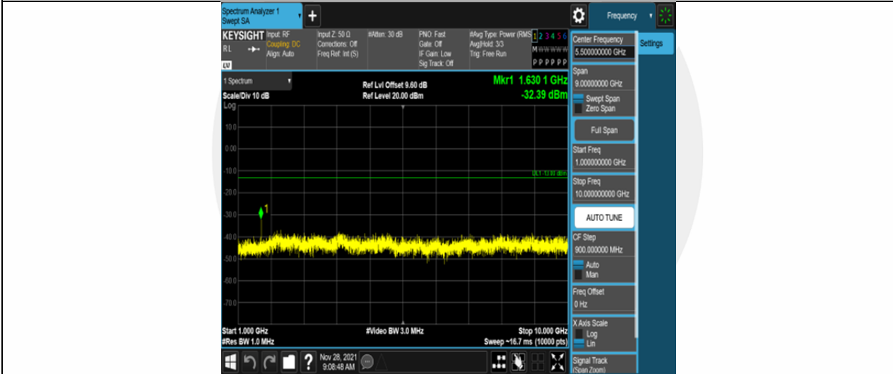
Band26-1.4MHz-QPSK-26697-6RB#0-Range2:1000~10000MHz
