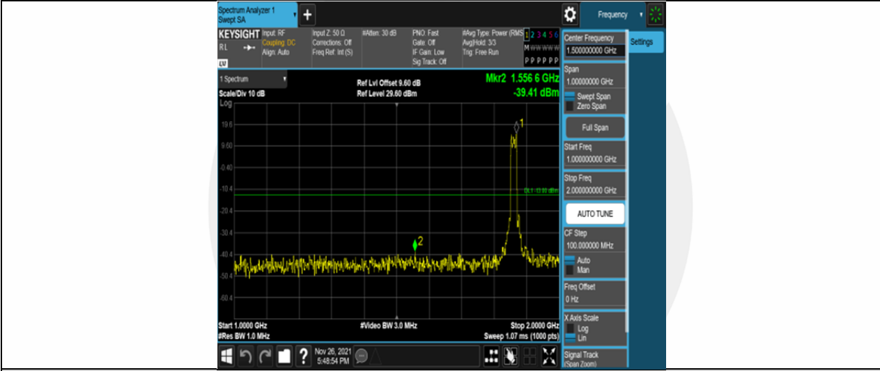
Band25-20MHz-QPSK-26140-100RB#0-Range2:1000~2000MHz
