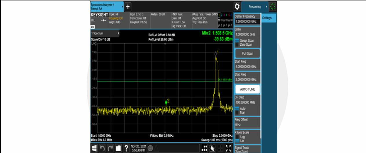
Band25-20MHz-16QAM-26365-100RB#0-Range2:1000~2000MHz
