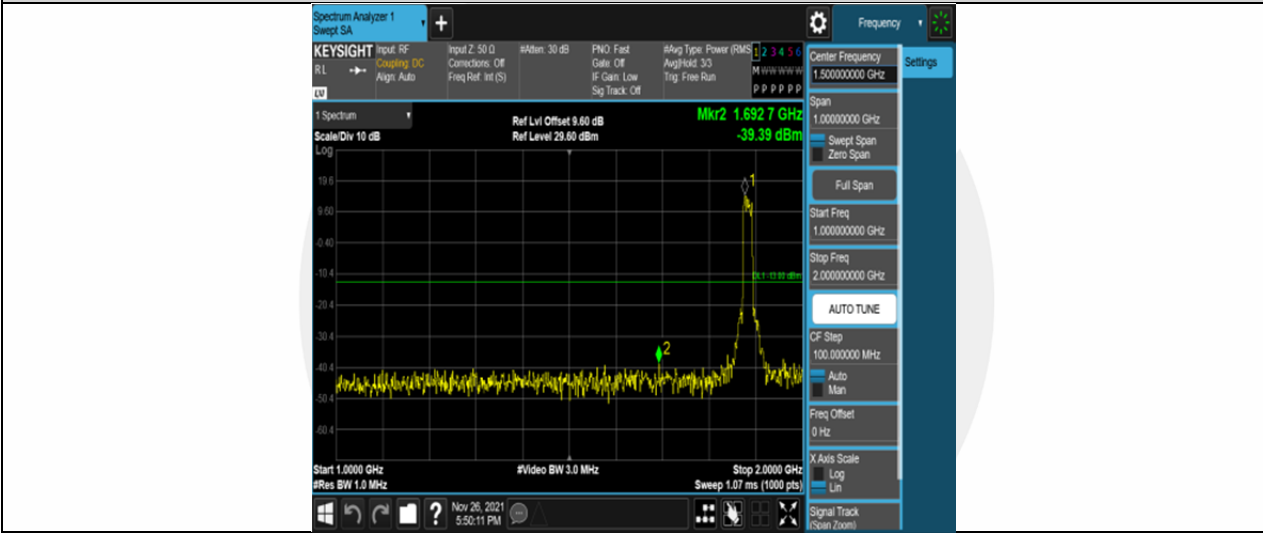
Band25-20MHz-QPSK-26365-100RB#0-Range2:1000~2000MHz
