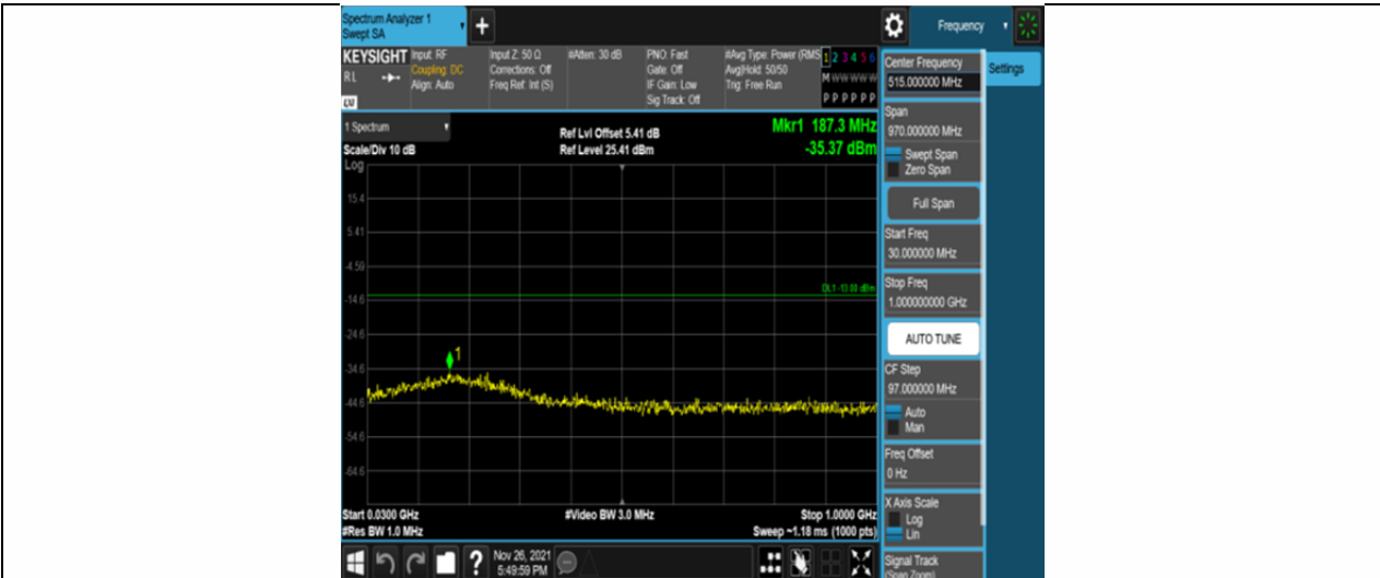
Band25-20MHz-QPSK-26365-100RB#0-Range1:30~1000MHz
