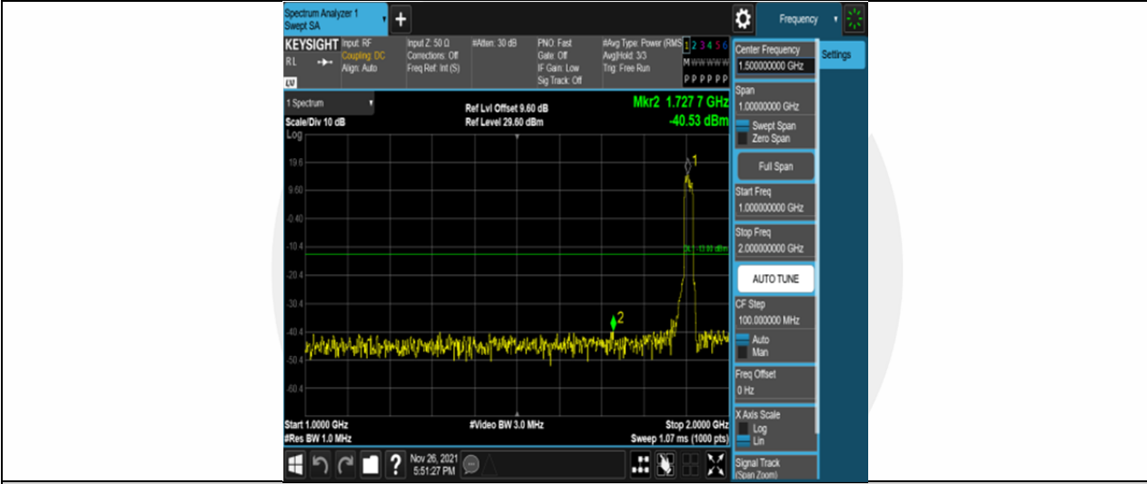
Band25-20MHz-QPSK-26590-100RB#0-Range2:1000~2000MHz
