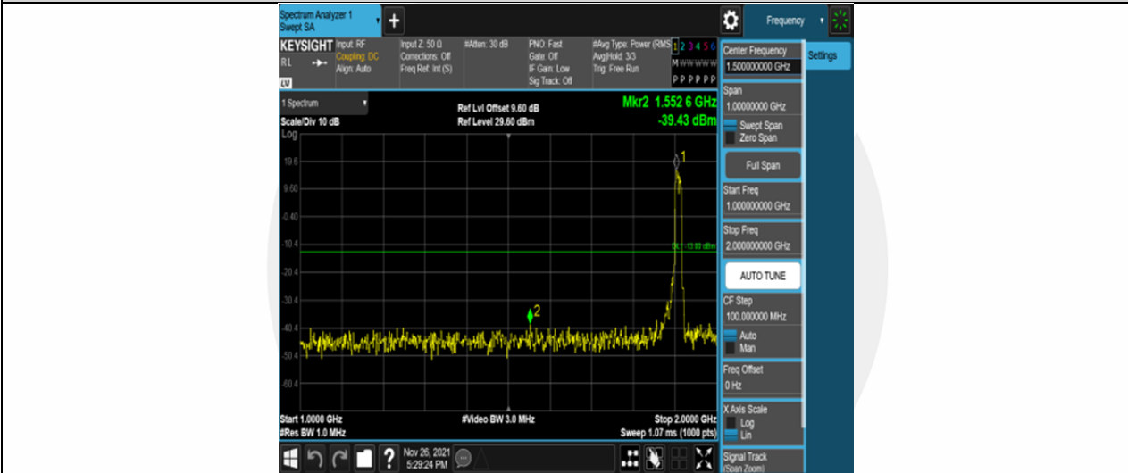
Band25-15MHz-QPSK-26615-75RB#0-Range2:1000~2000MHz
