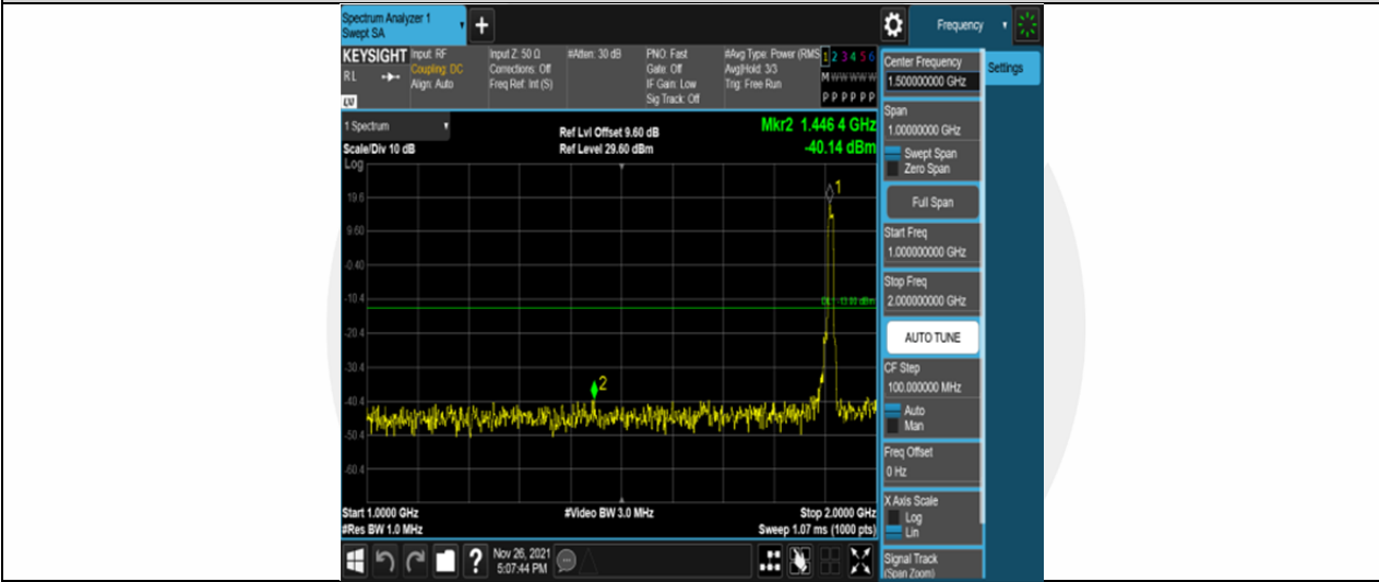
Band25-10MHz-QPSK-26640-50RB#0-Range2:1000~2000MHz
