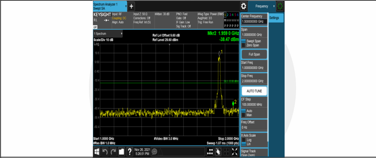
Band25-15MHz-QPSK-26115-75RB#0-Range2:1000~2000MHz
