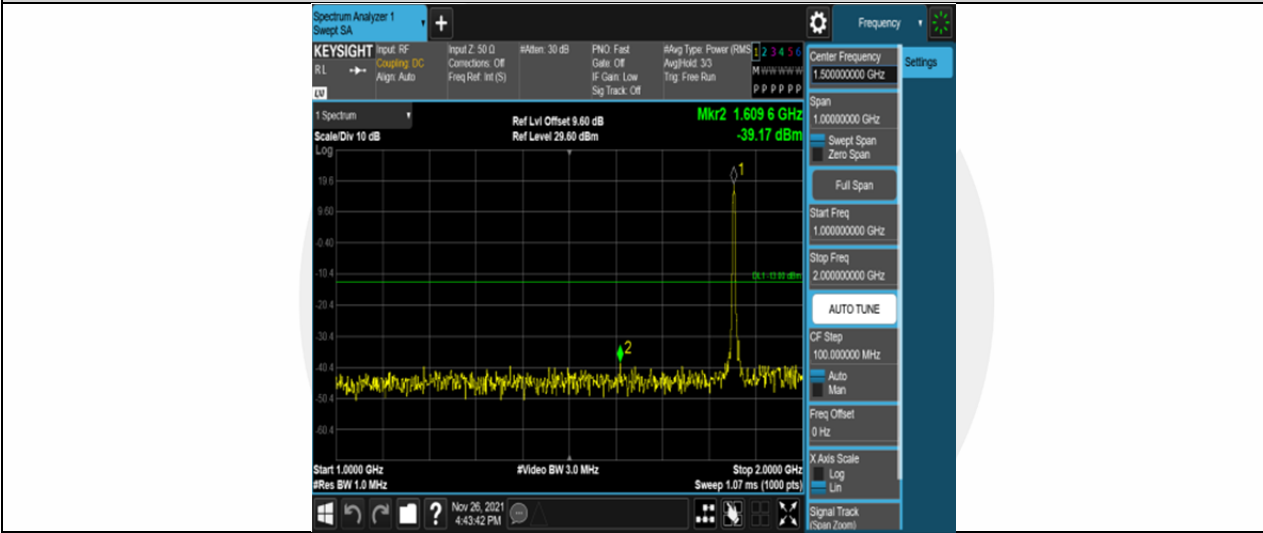
Band25-5MHz-QPSK-26065-25RB#0-Range2:1000~2000MHz
