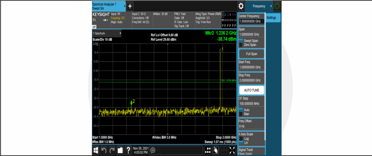
Band25-1.4MHz-16QAM-26365-6RB#0-Range2:1000~2000MHz
