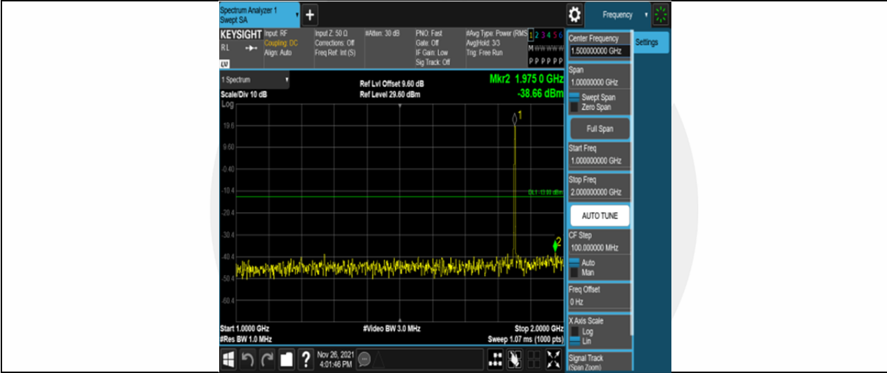
Band25-1.4MHz-16QAM-26047-6RB#0-Range2:1000~2000MHz
