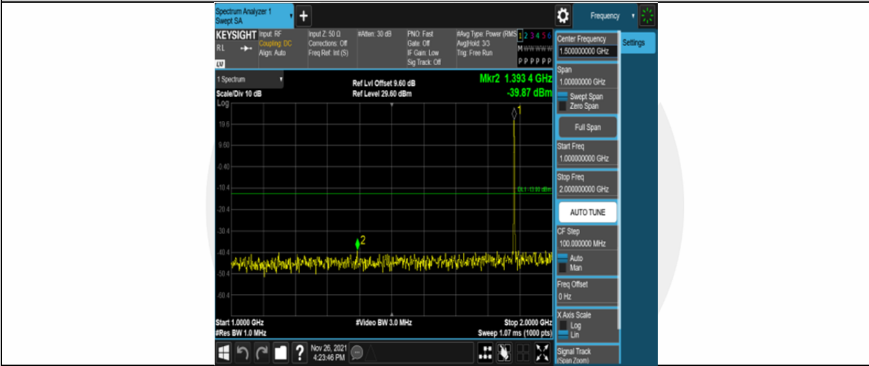
Band25-3MHz-16QAM-26365-1RB#0-Range2:1000~2000MHz
