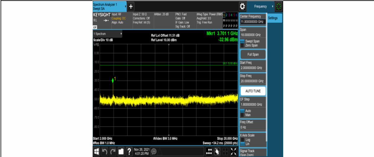
Band25-1.4MHz-QPSK-26047-6RB#0-Range3:2000~20000MHz
