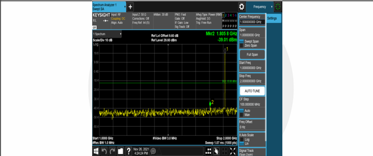
Band25-3MHz-QPSK-26675-1RB#0-Range2:1000~2000MHz
