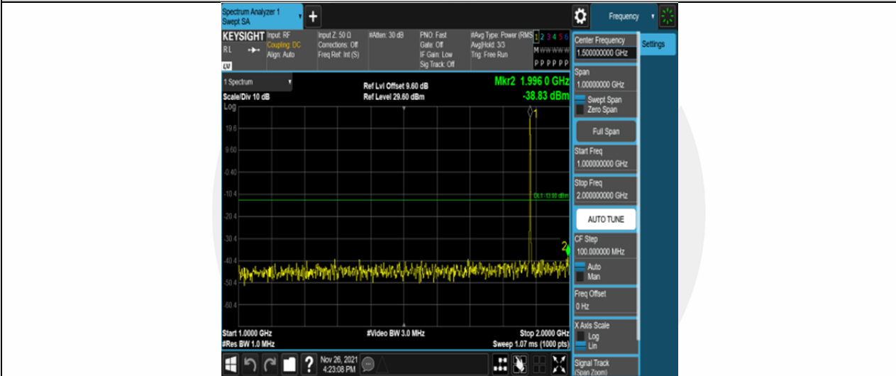
Band25-3MHz-QPSK-26365-1RB#0-Range2:1000~2000MHz
