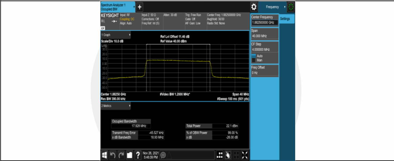
Band25-20MHz-16QAM-26365-100RB#0
