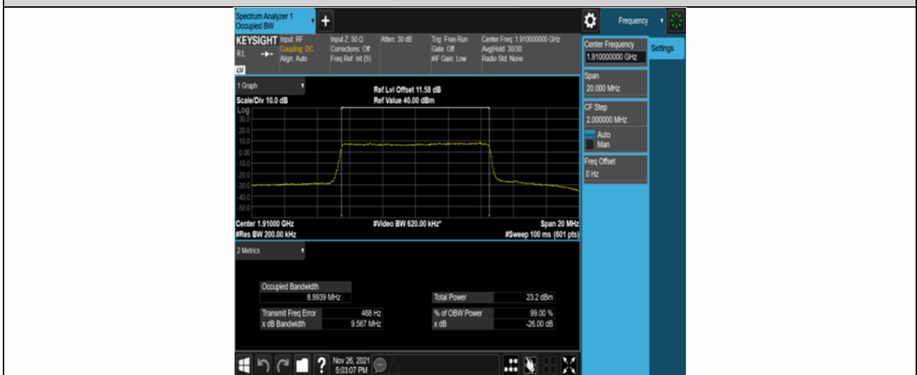
Band25-10MHz-QPSK-26640-50RB#0
