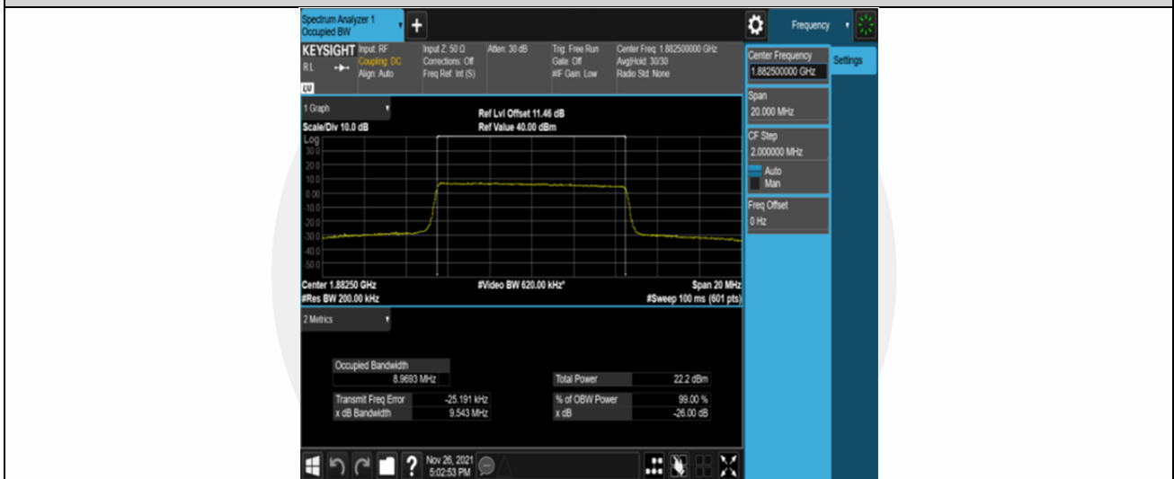
Band 25-10MHz-16QAM-26365-50RB#0
