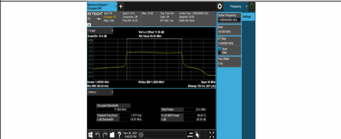
Band25-20MHz-QPSK-26590-100RB#0
