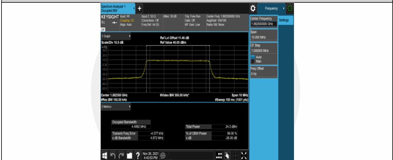
Band25-5MHz-QPSK-26365-25RB#0
