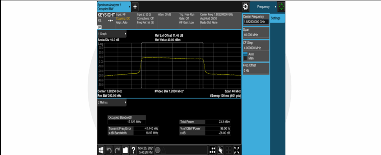
Band25-20MHz-QPSK-26365-100RB#0
