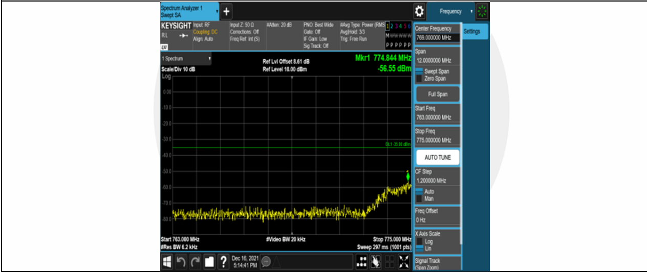
Band13-5MHz-QPSK-23205-25RB#0-Range3:763~775MHz
