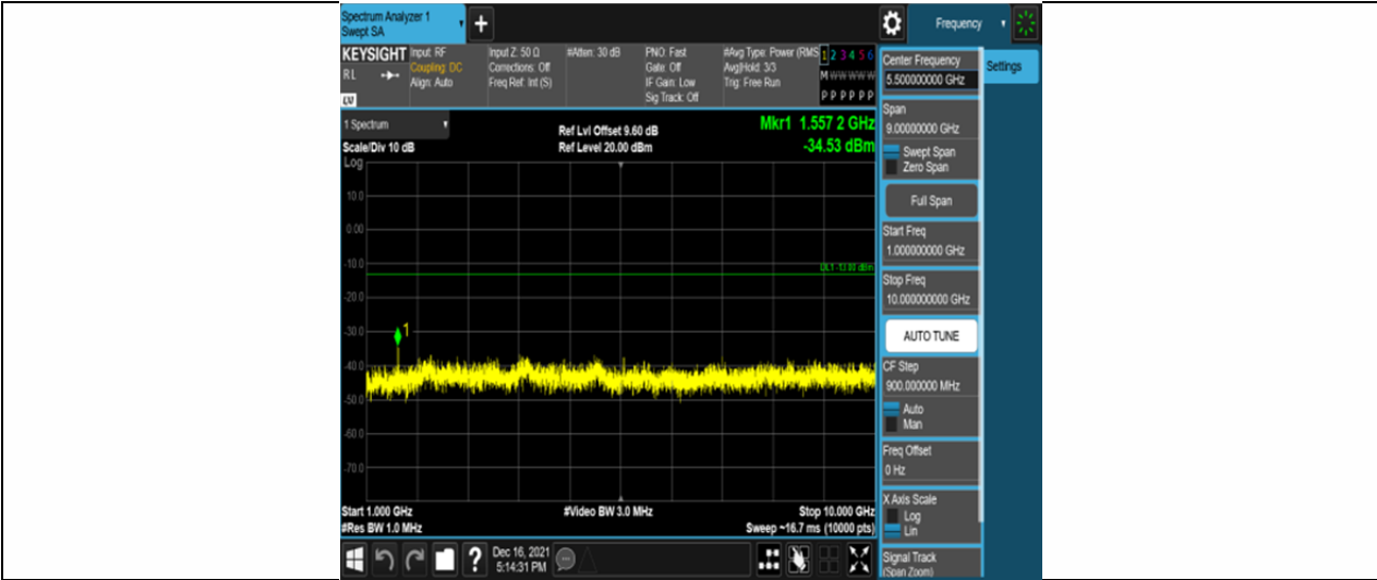
Band13-5MHz-QPSK-23205-25RB#0-Range2: 1000~10000MHz
