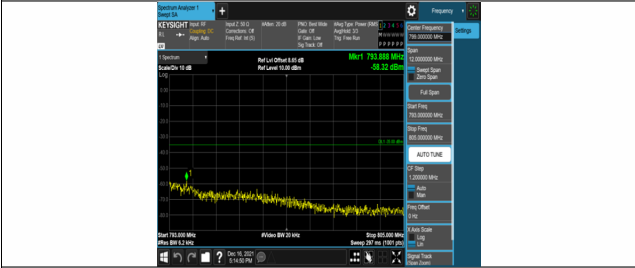
Band13-5MHz-QPSK-23205-25RB#0-Range4:793~805MHz
