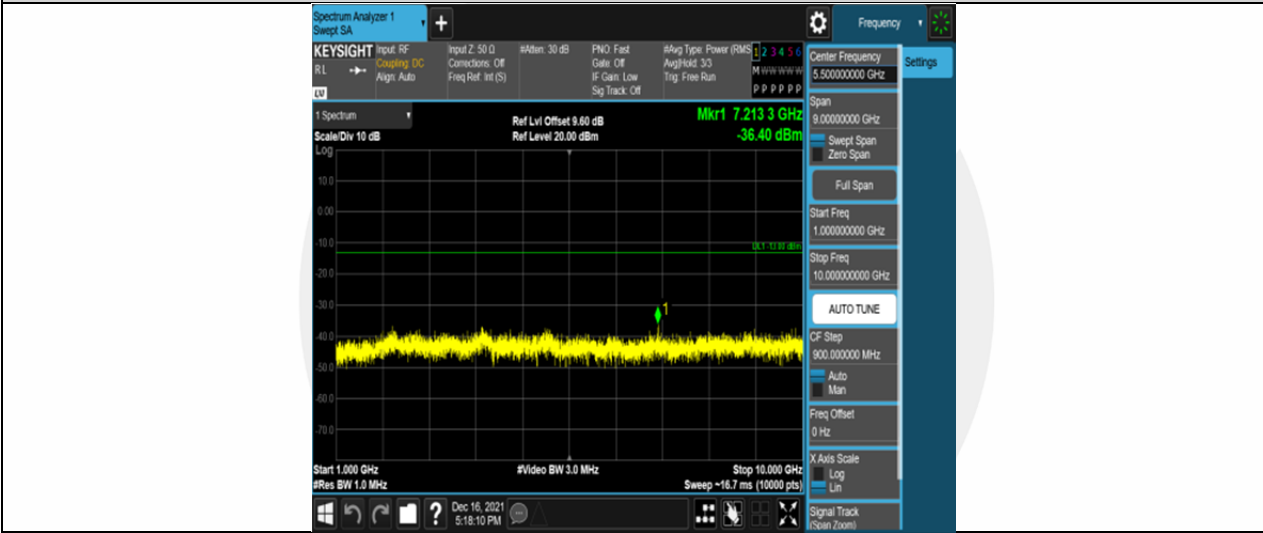
Band13-5MHz-QPSK-23255-25RB#0-Range2:1000~10000MHz
