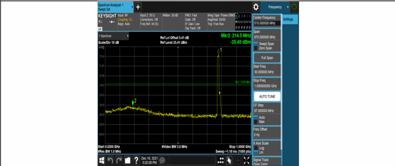
Band13-5MHz-QPSK-23230-25RB#0-Range1:30~1000MHz
