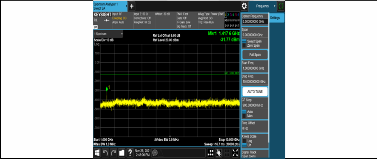
Band12-10MHz-QPSK-23130-50RB#0-Range2:1000~10000MHz
