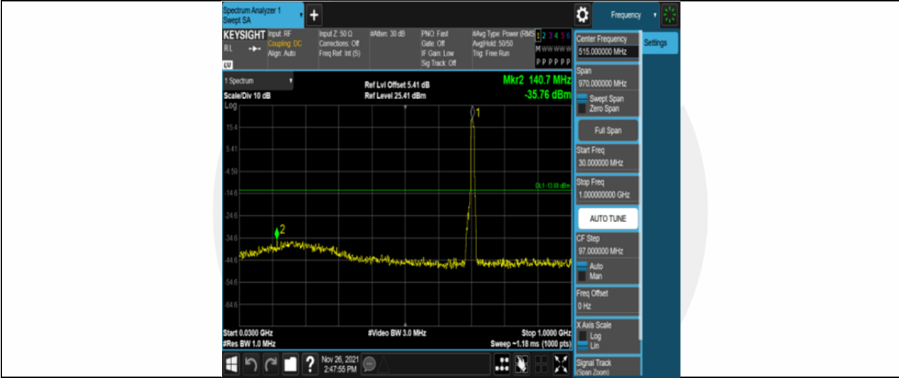
Band12-10MHz-QPSK-23130-50RB#0-Range1:30~1000MHz
